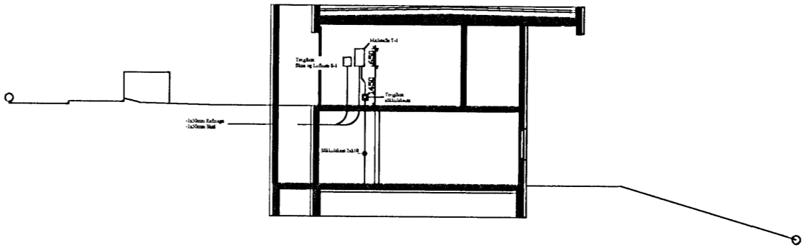
ÞVERSNIÐ FURUÁS 12
