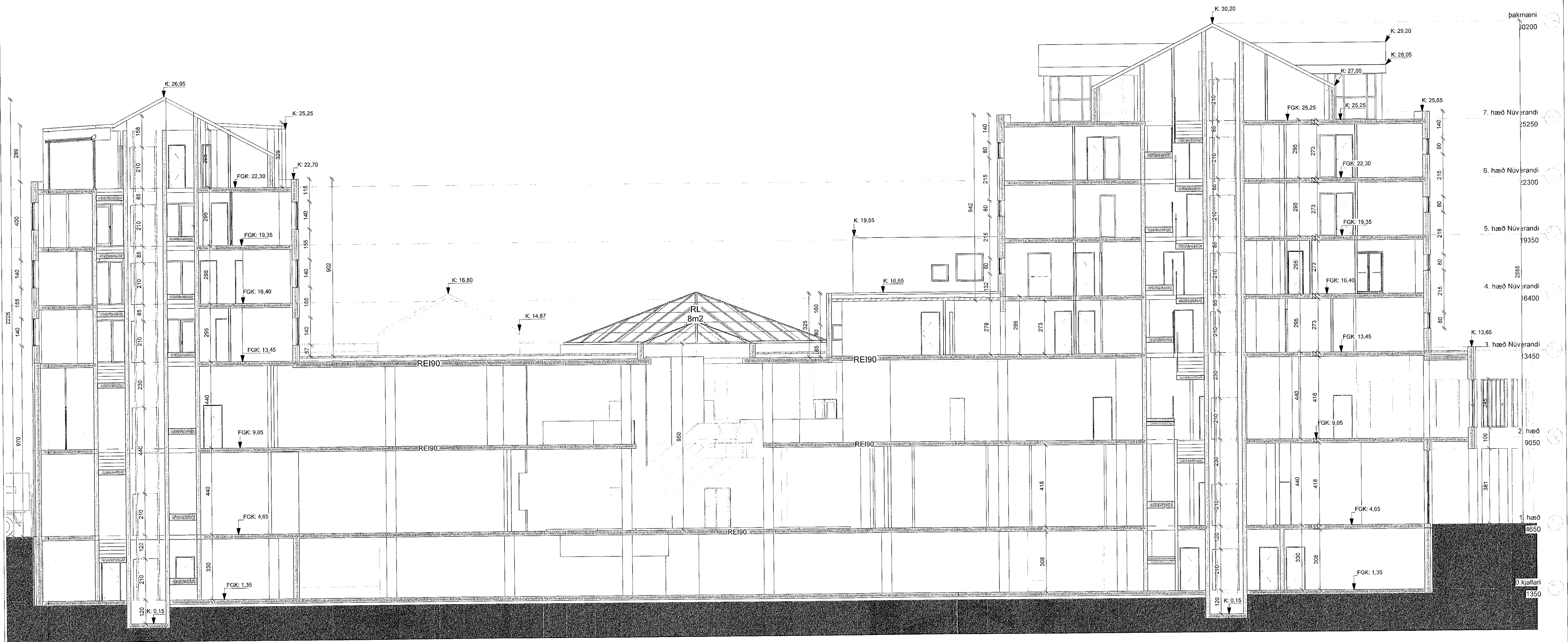
Sneiðing G-G 1:100
