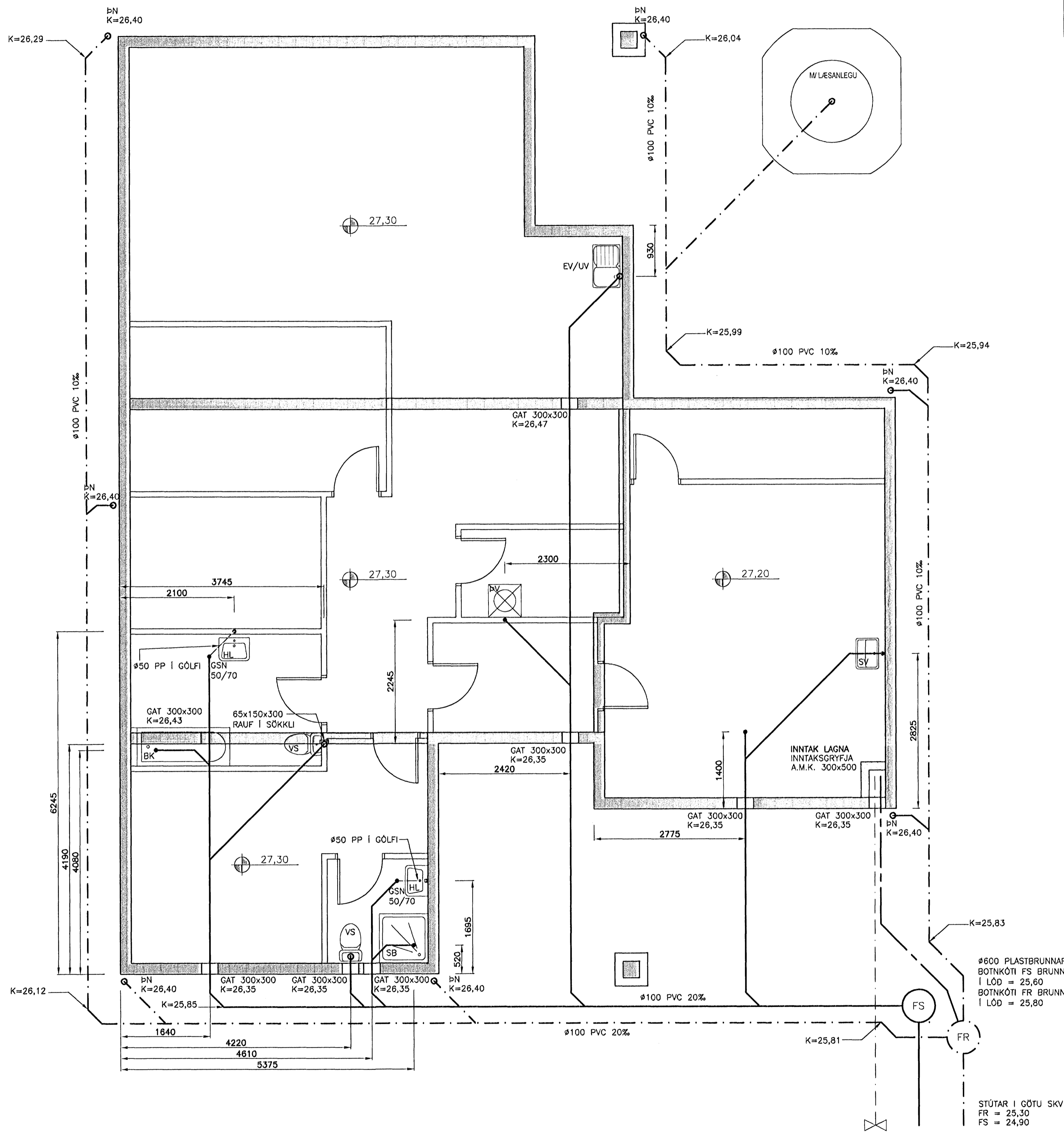
GRUNNMYND FRÄRENNSLISLAGNA MKV. 1:50
