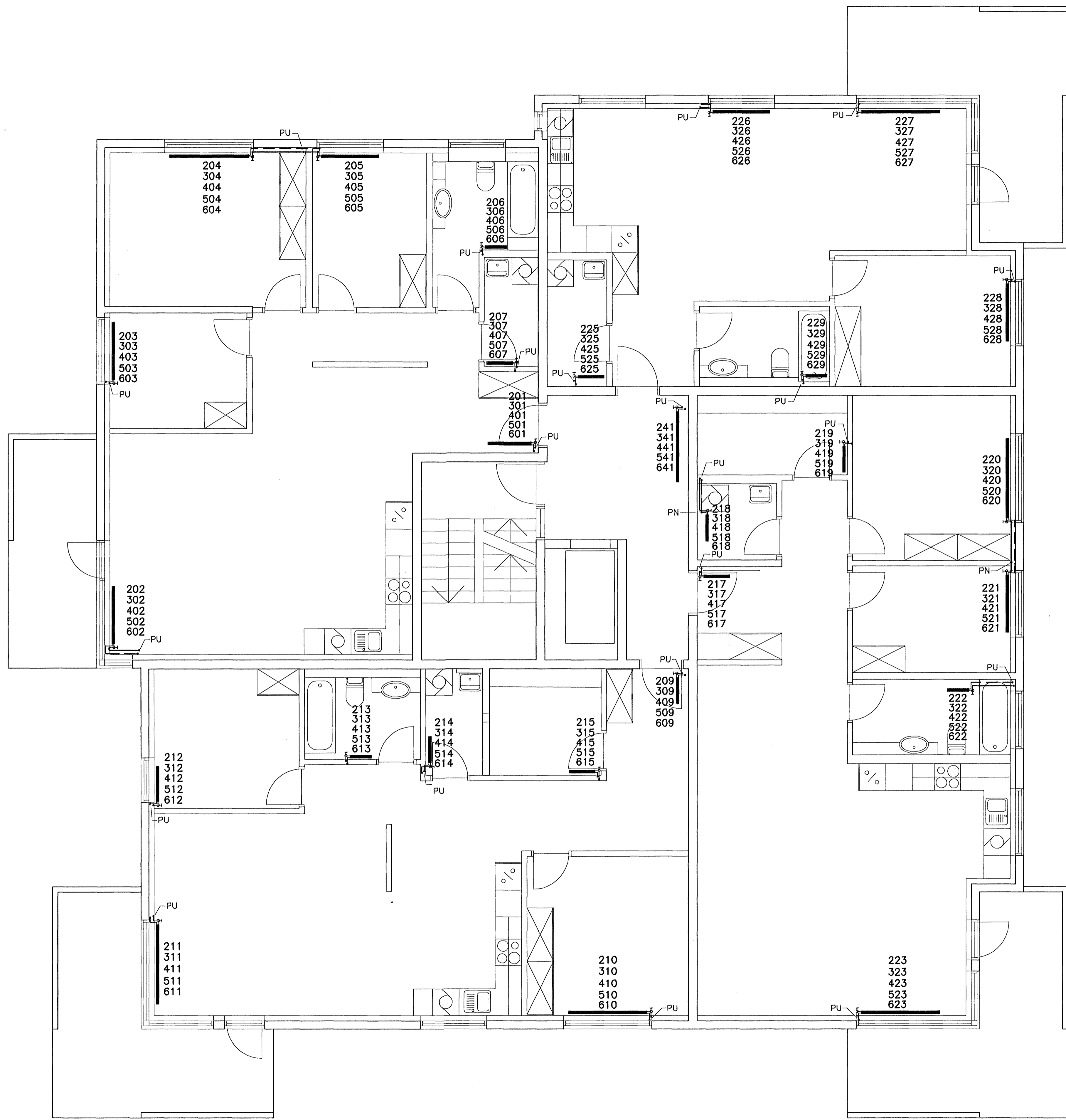
GRUNNMYND 2-6.HÆÐ. 1:50
