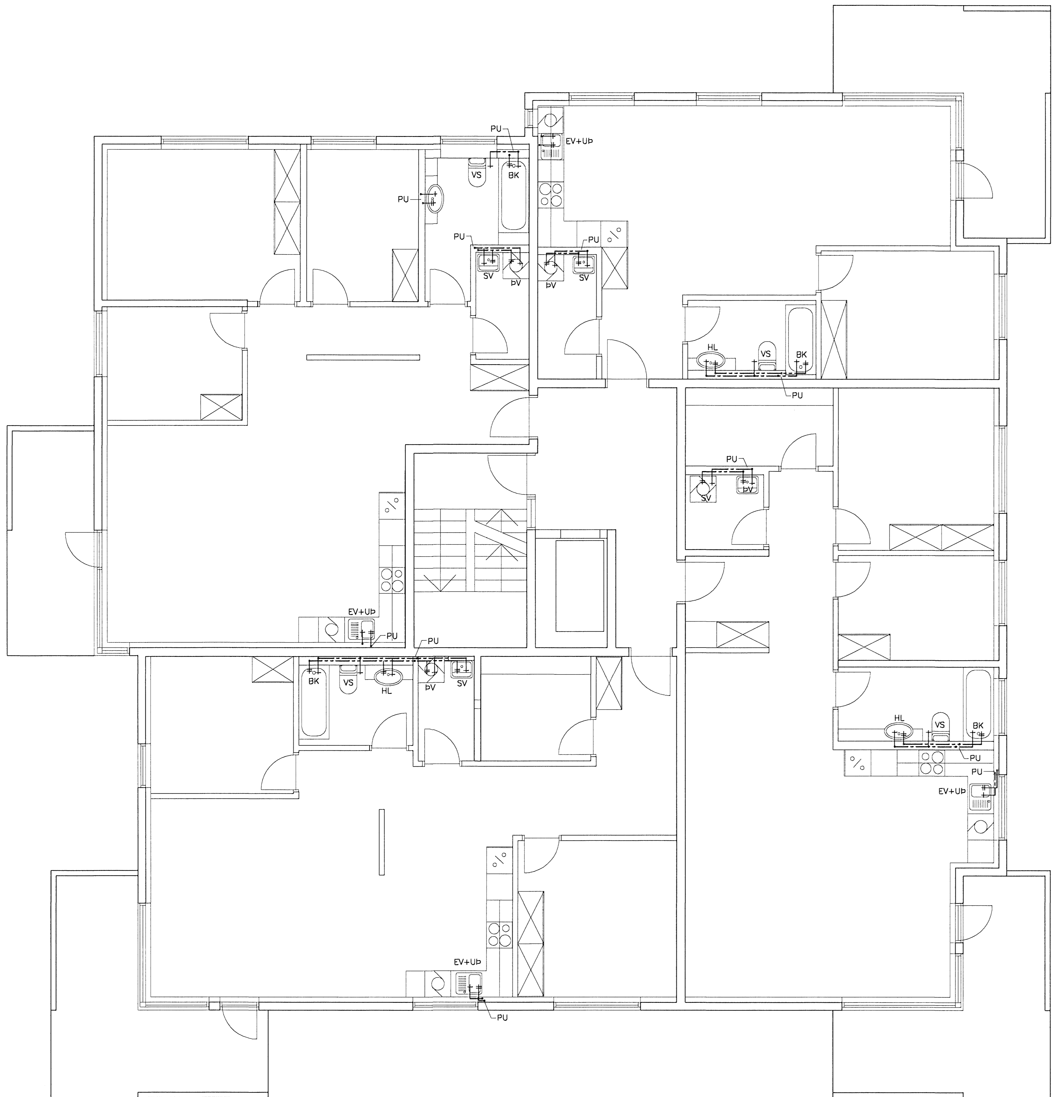
GRUNNMYND 3-6.HÆÐ, 1:50
