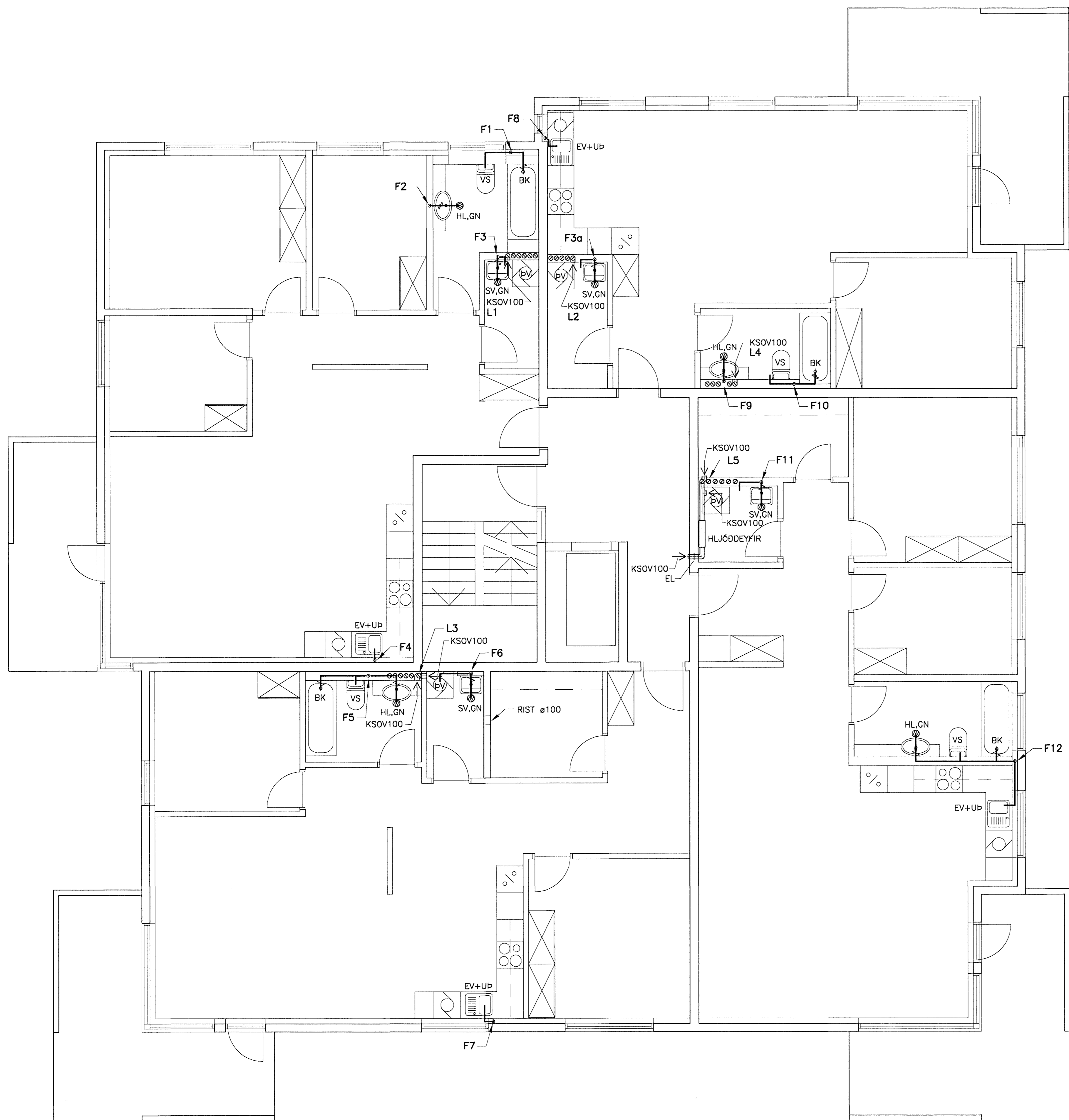
GRUNNMYND 6.HÆÐ. 1:50
