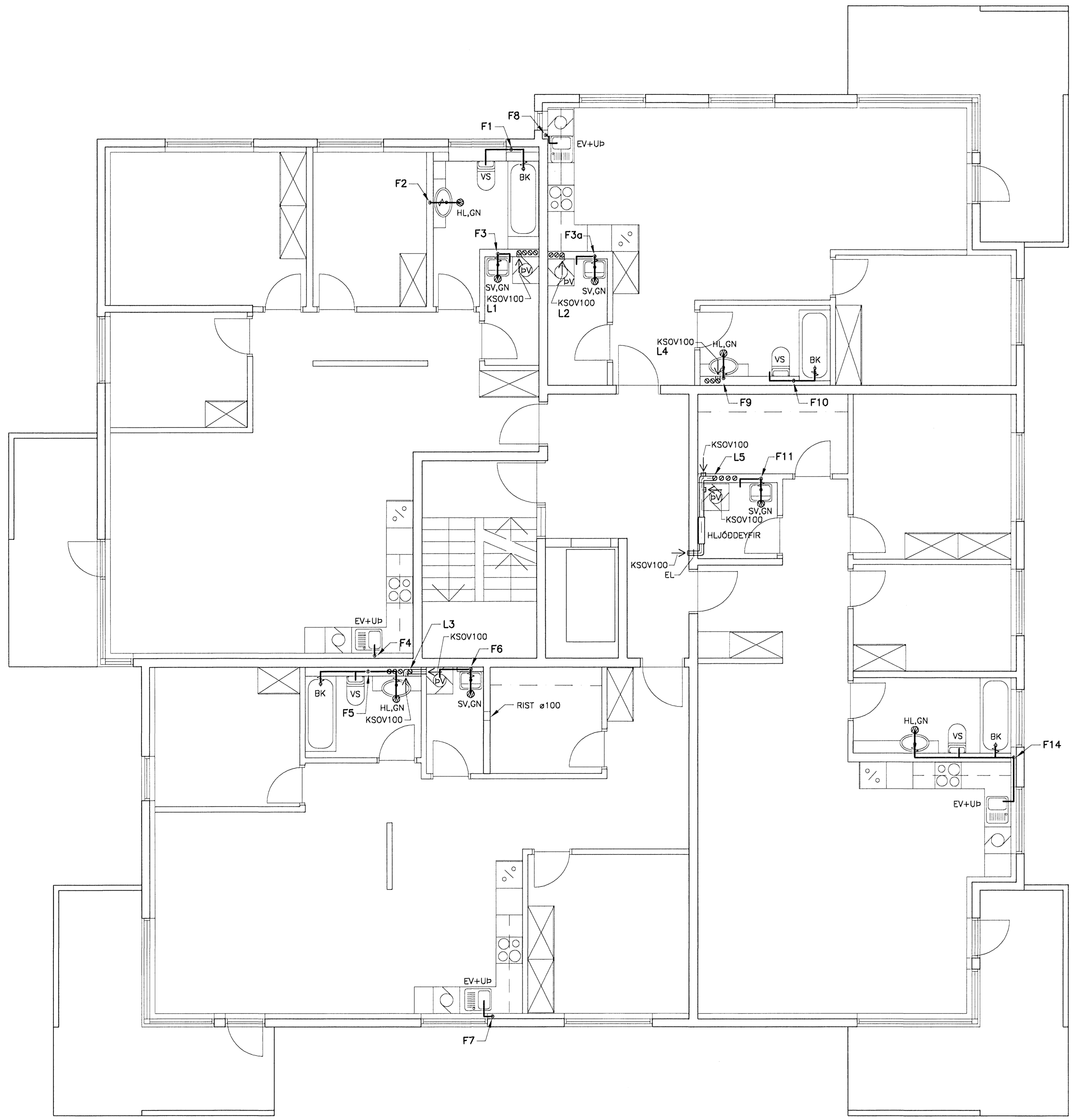
GRUNNMYND 4.HÆÐ, 1:50
