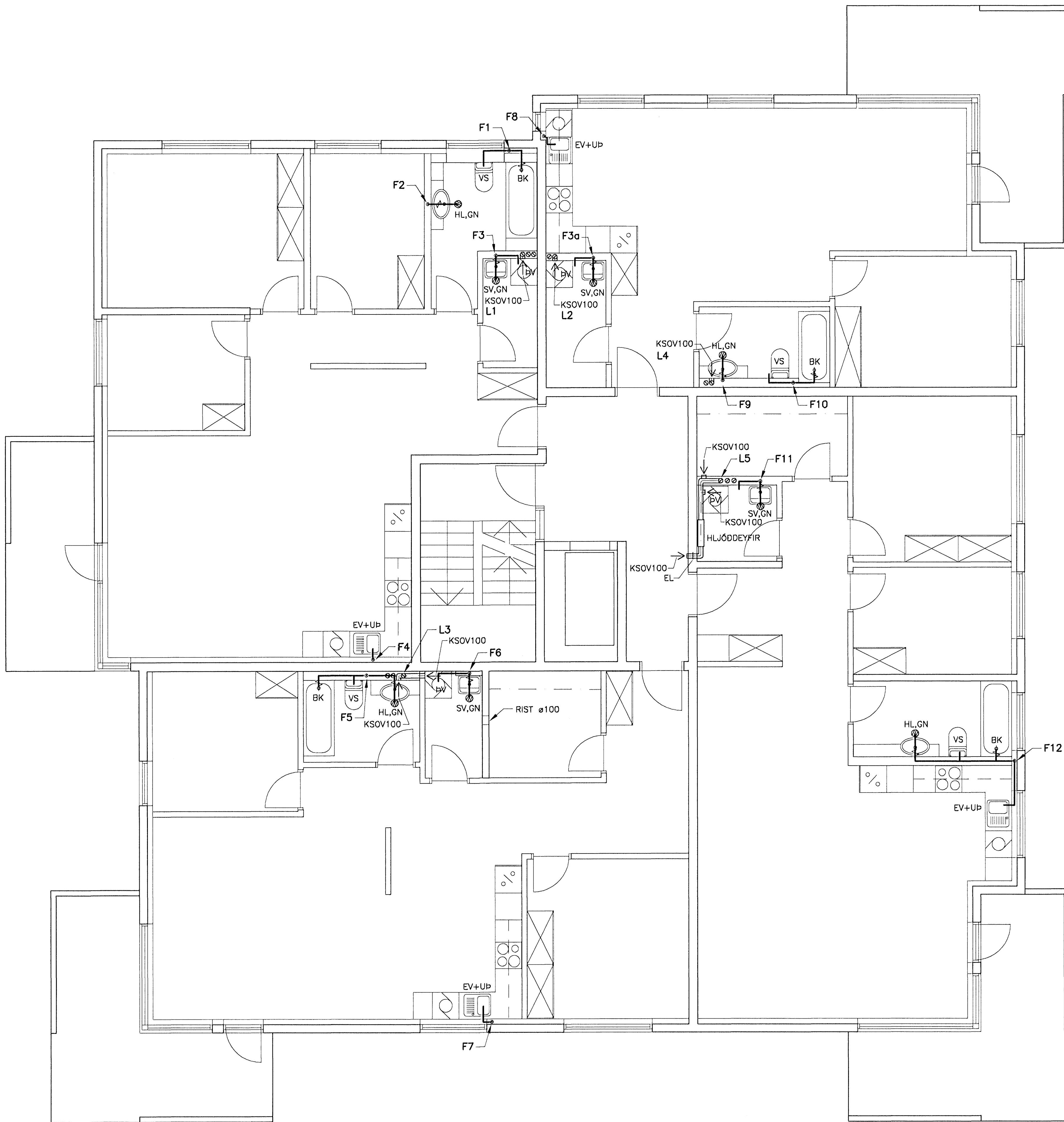
GRUNNMYND 3.HÆÐ, 1:50
