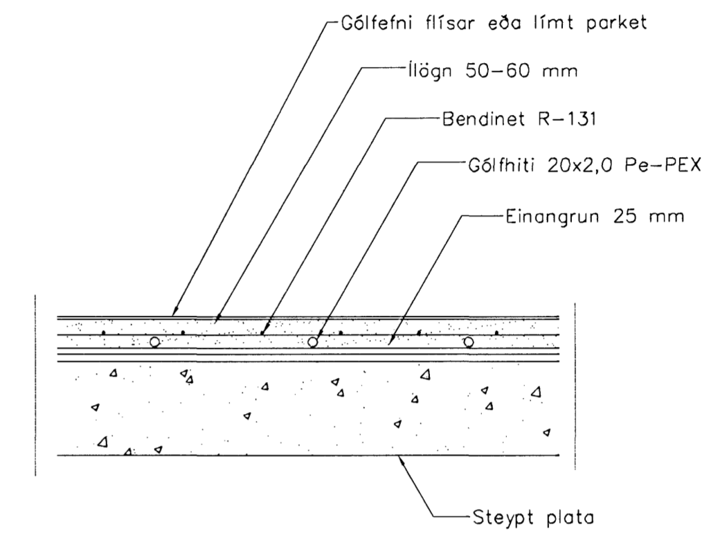
Gólfhiti snið, 1:10
