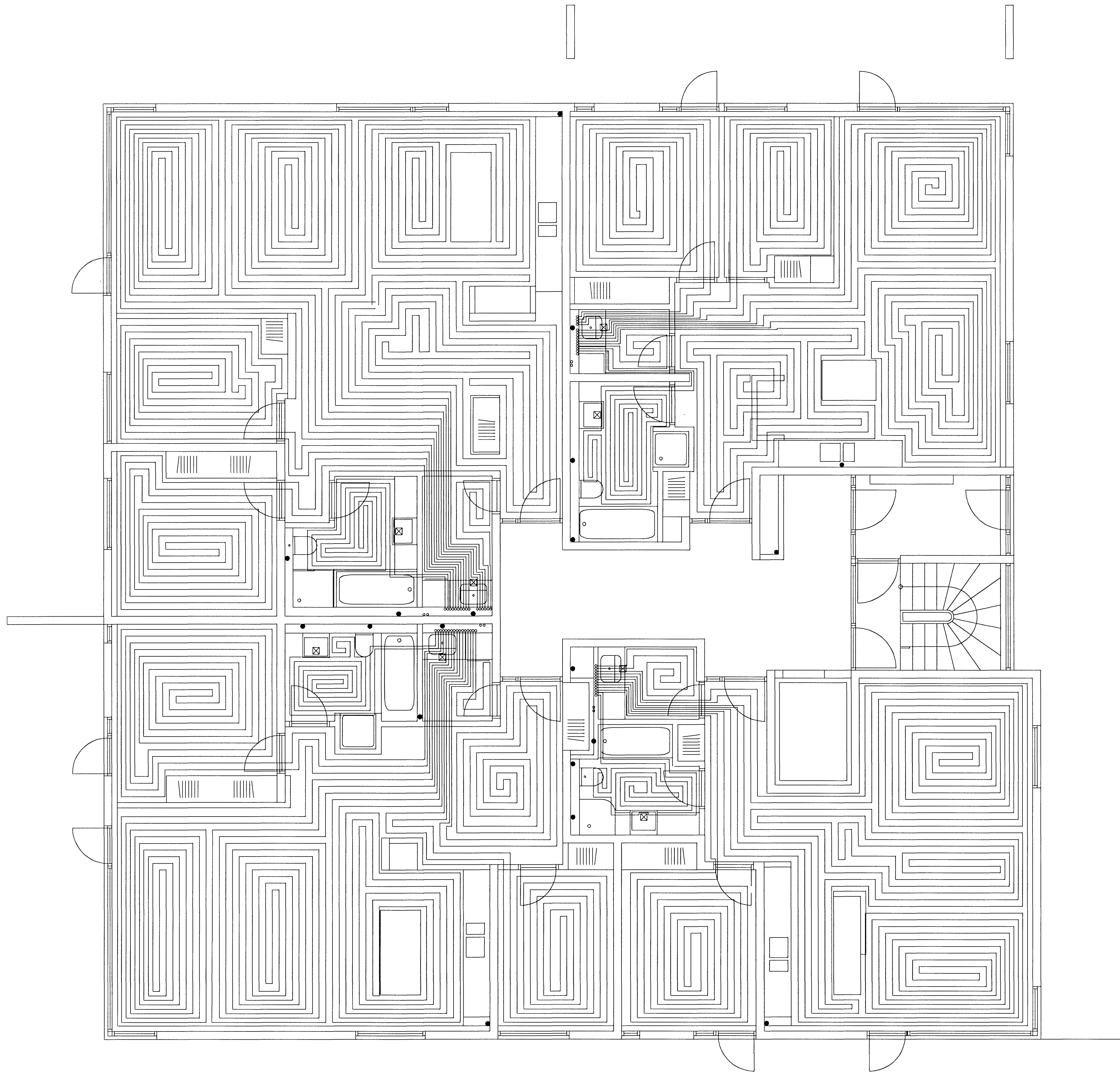
GRUNNMYND 1 HÆÐAR 1:50
