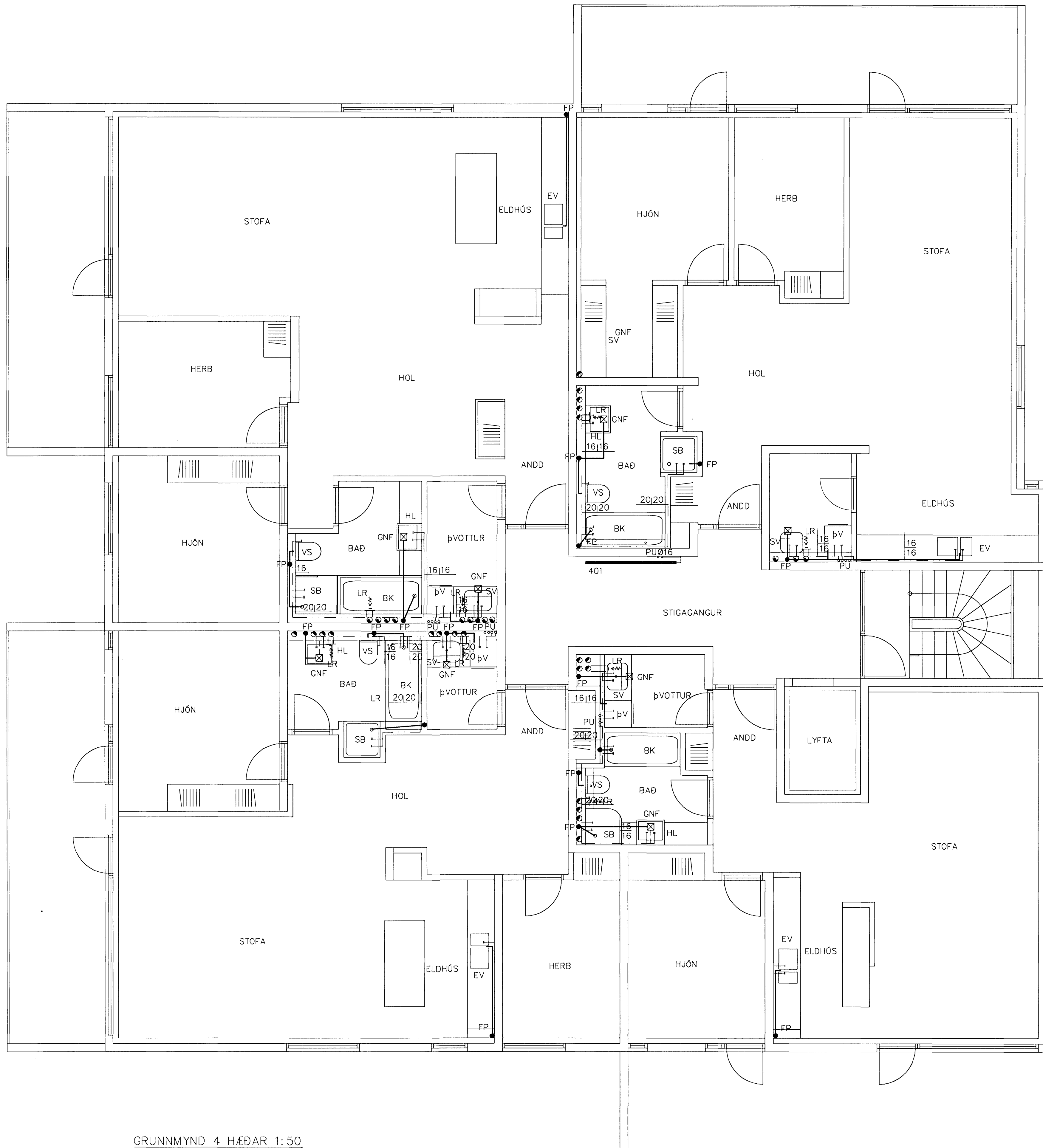
GRUNNMYND 4 HÆÐAR 1:50
