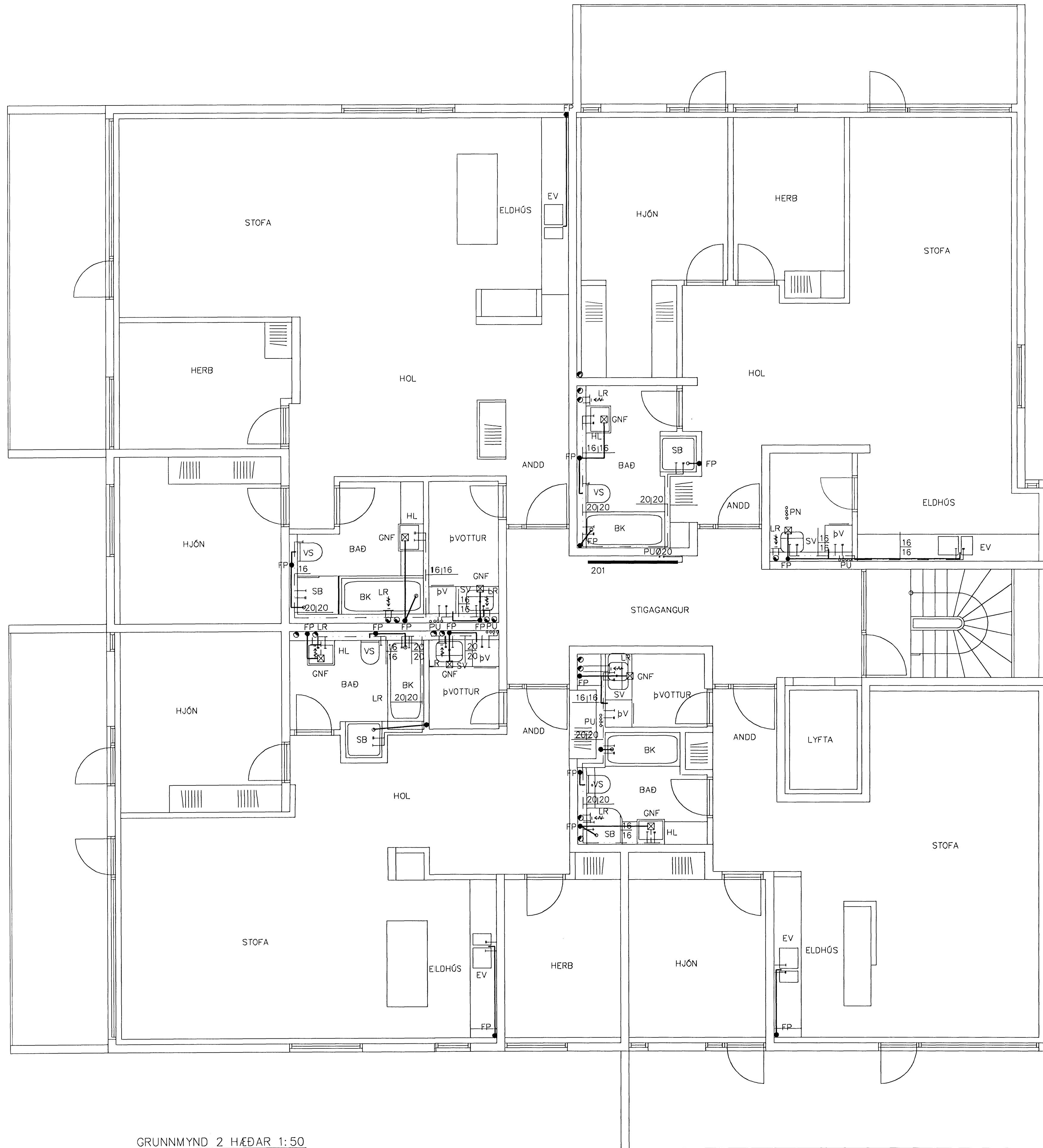
GRUNNMYND 2. HÆÐAR 1:50
