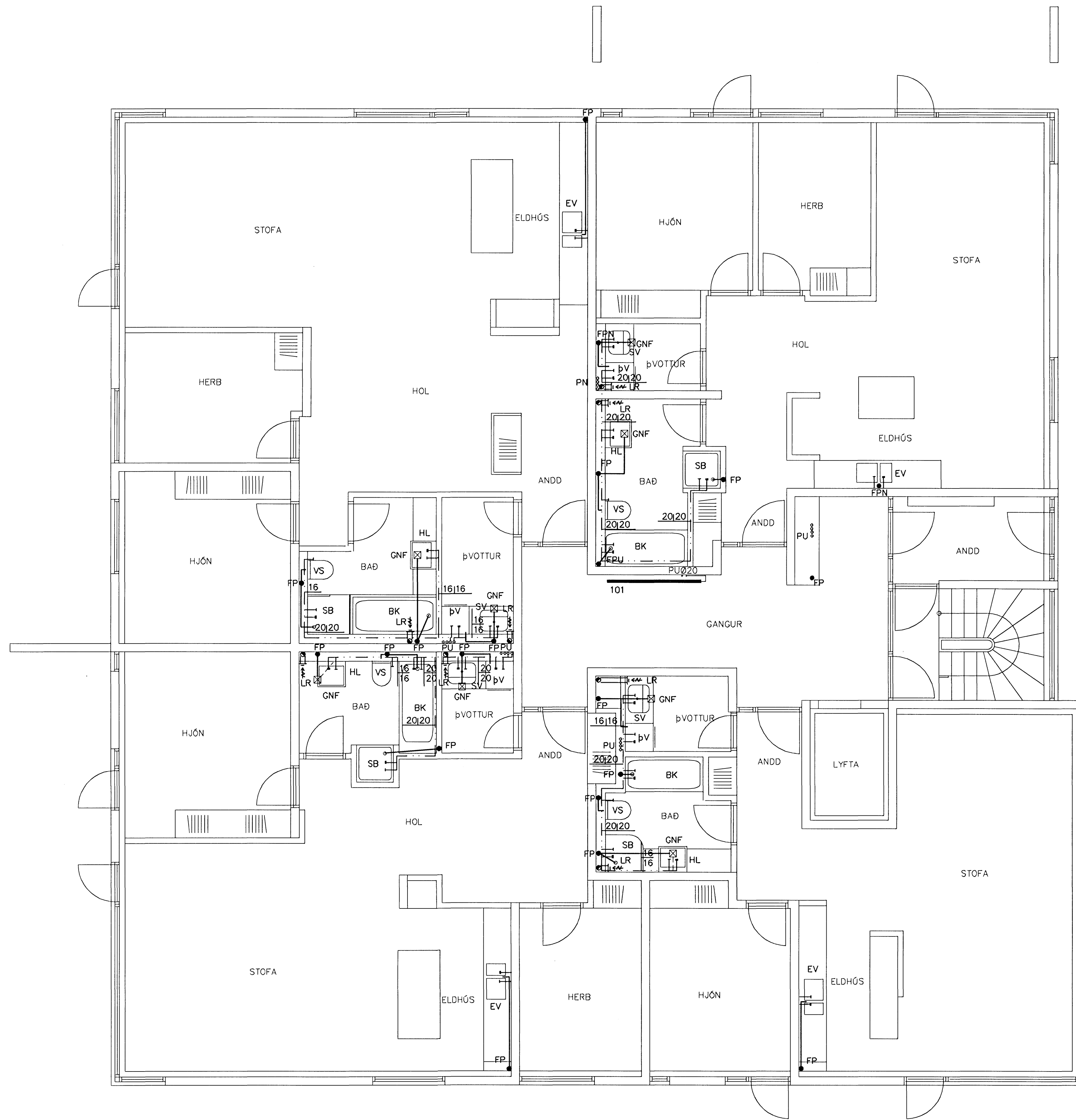
GRUNNMYND 1 HÆÐAR 1:50
