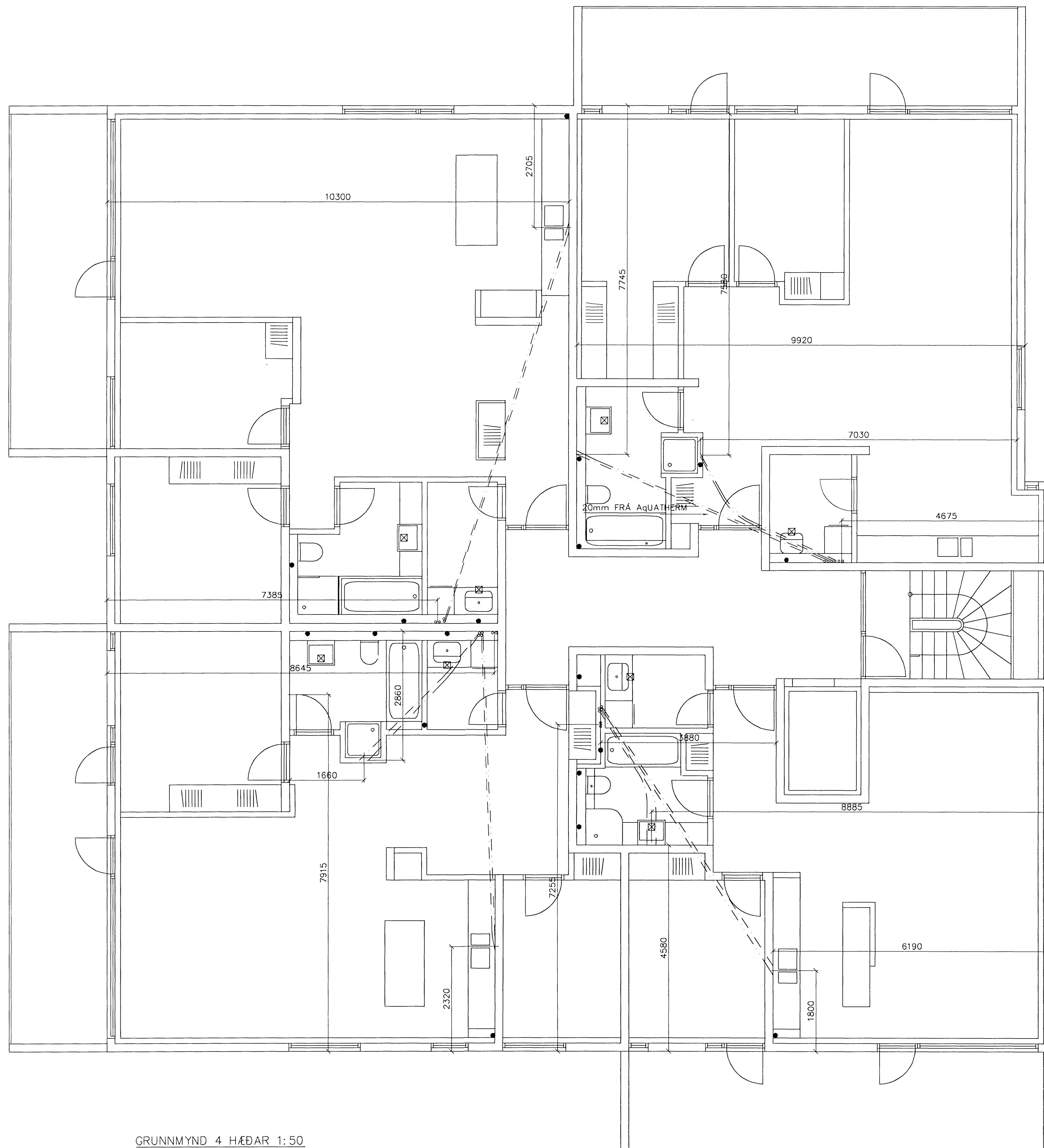
GRUNNMYND 4 HÆÐAR 1:50
