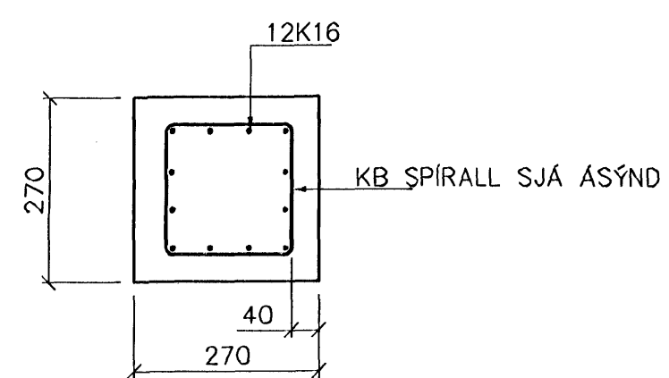
SNÍÐ A 1:10
