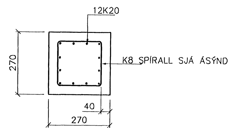
SNÍÐ B 1:10
