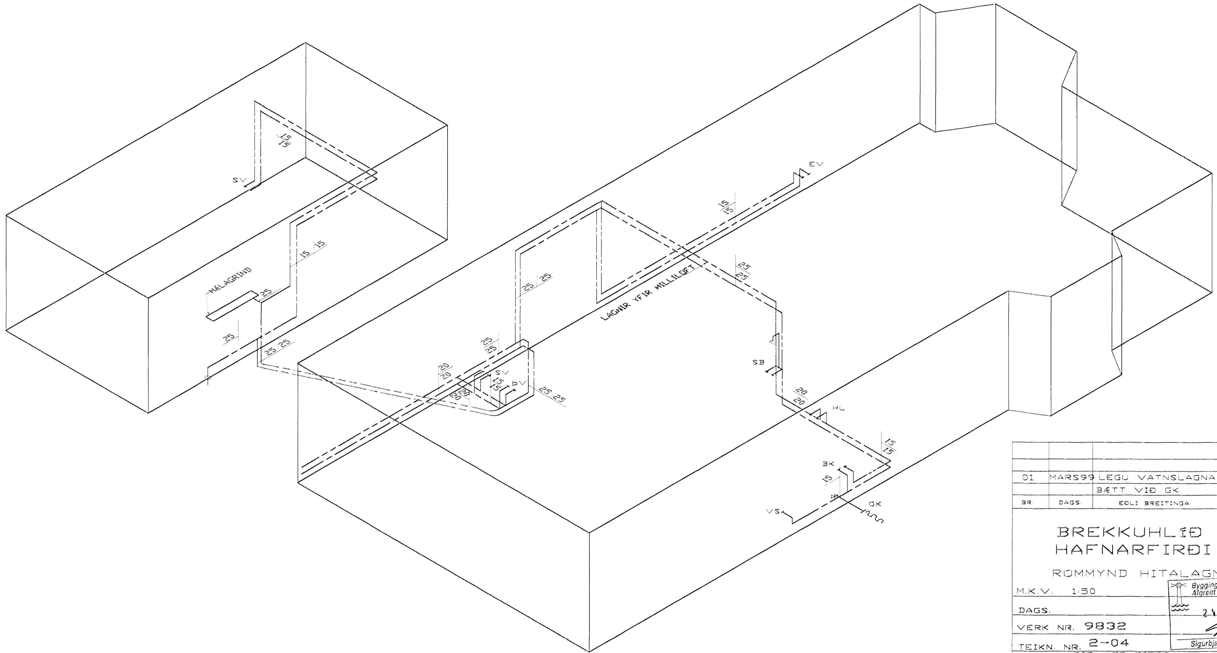
RÜMMYND VATNSLAGNA 1:50
