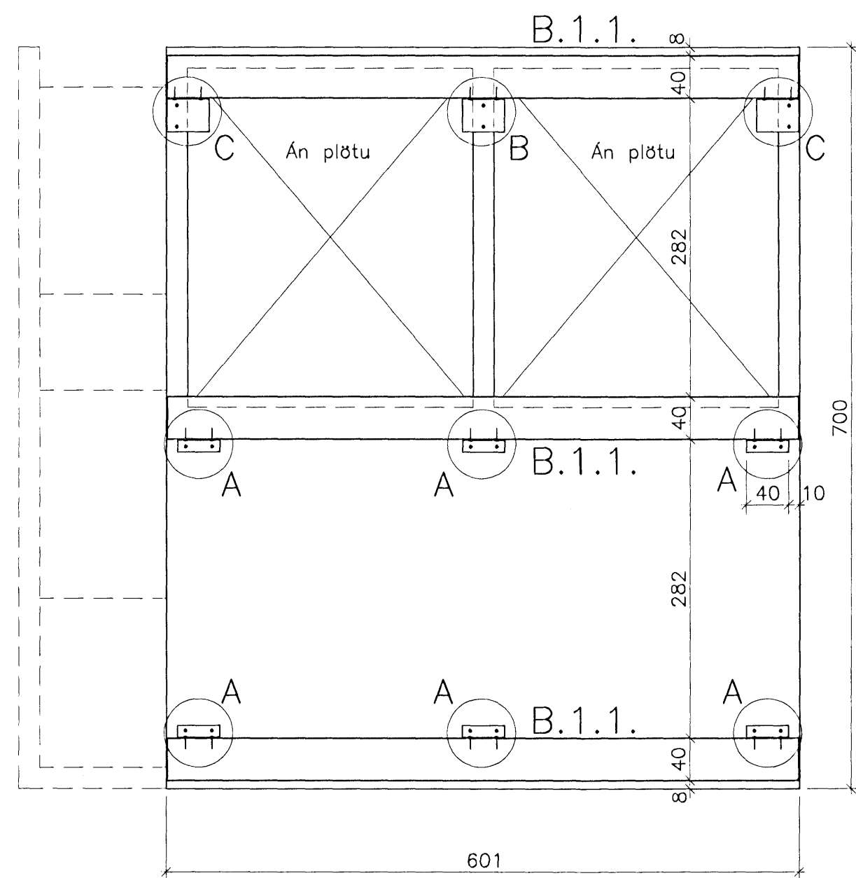
Undirstöðubitar í starfsmannaástaðu Grunnmynd 1:50
