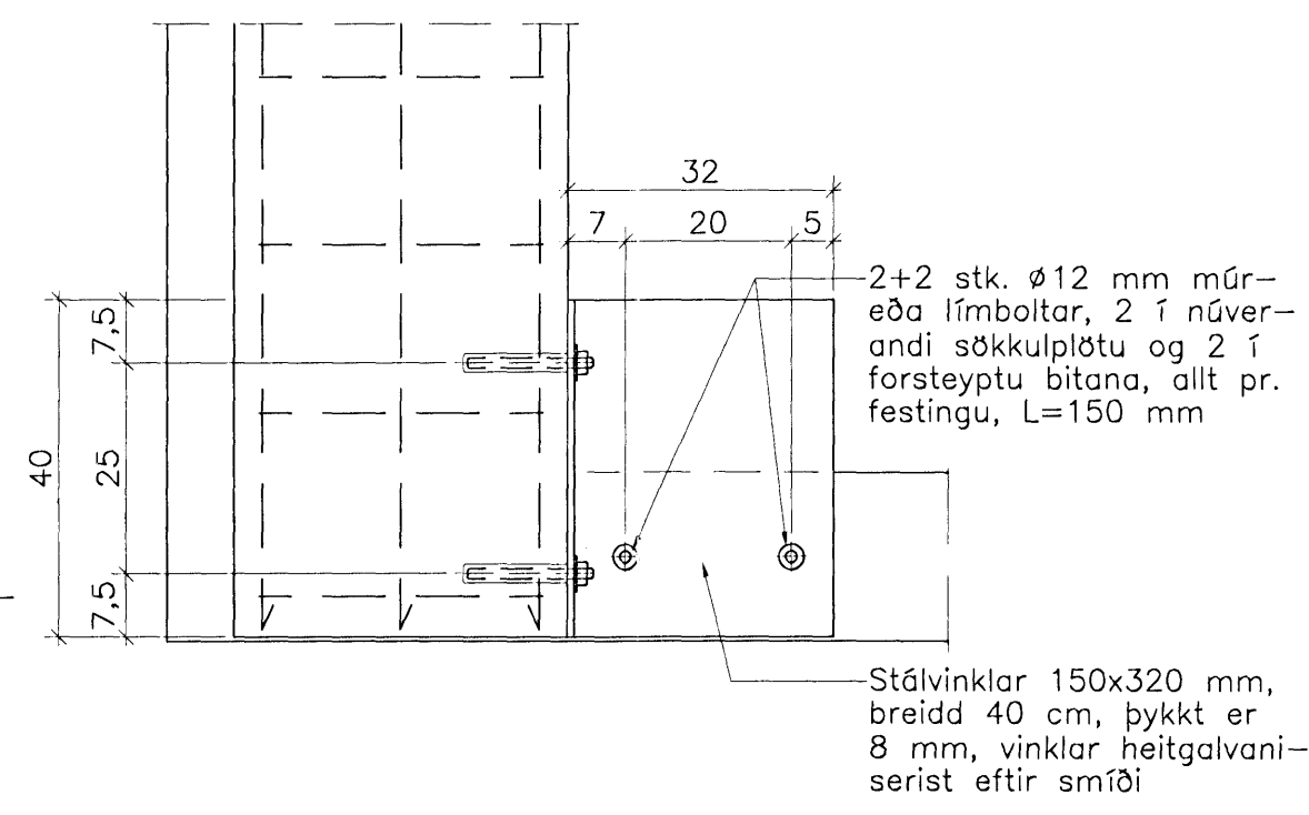
Sérmynd C 1:10 2. stk.
