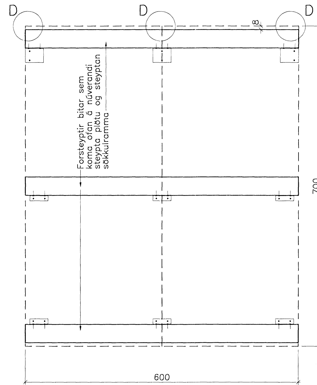
Gámafestingar í starfsmannaástaðu Grunnmynd 1:50
