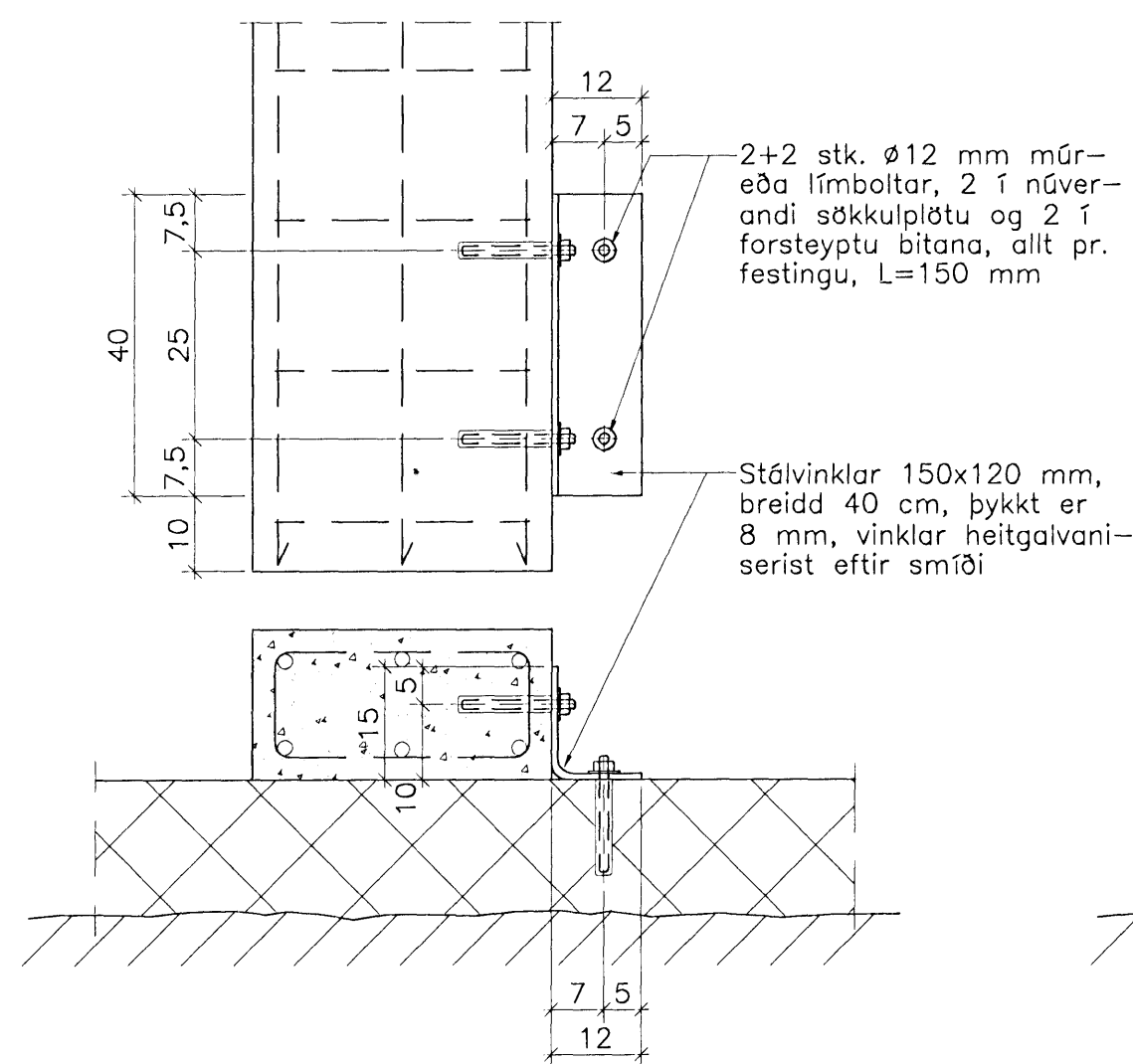
Sérmynd A 1:10 6. stk.
