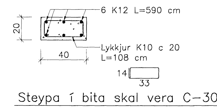
Snið í B.1.1. 1:20 L=600 cm, 3. stk.
