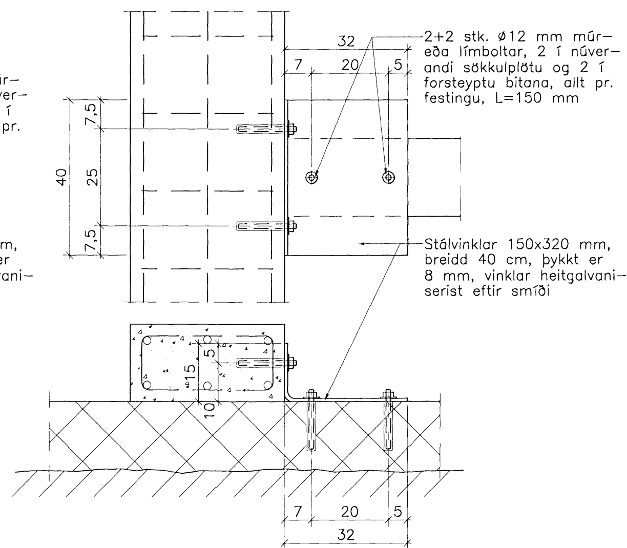
Sérmynd B 1:10 1. stk.
