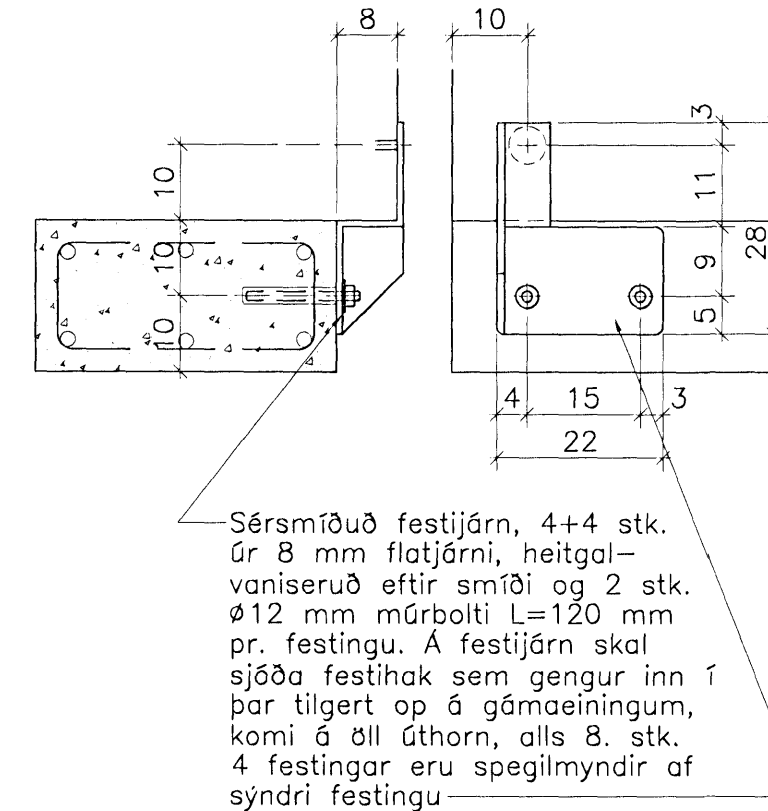
Sérmynd D 1:10 4+4. stk.
