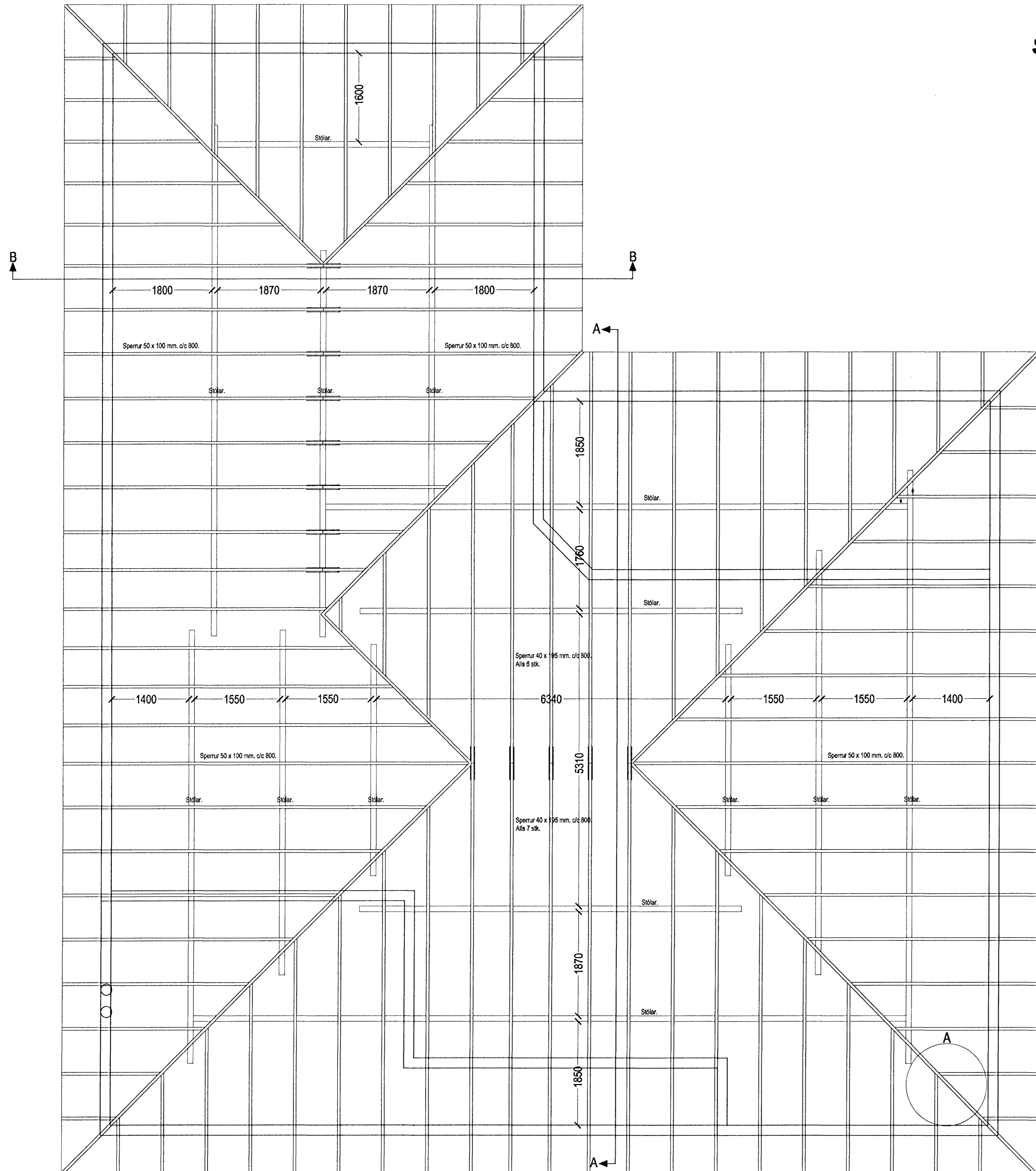
GRUNNMYND ÞAKVIRKI, MKV. 1:50.
