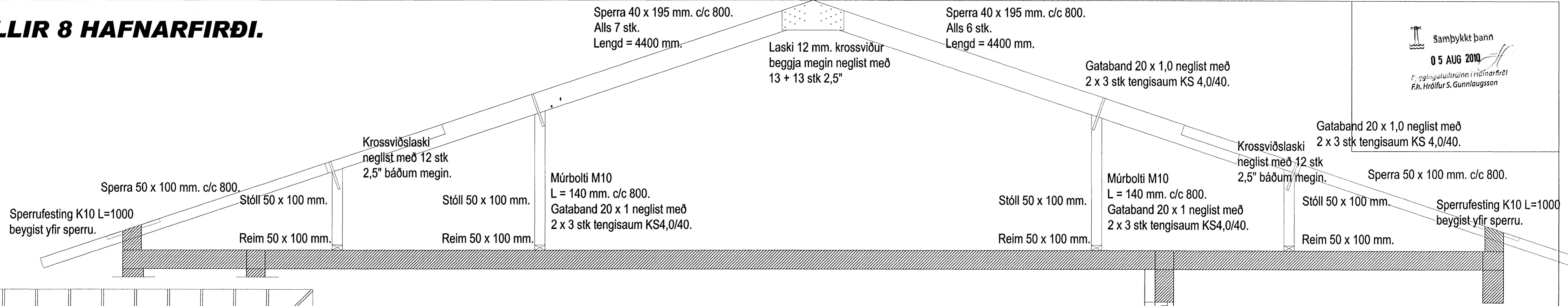
SNID A - A MKV. 1:20.
