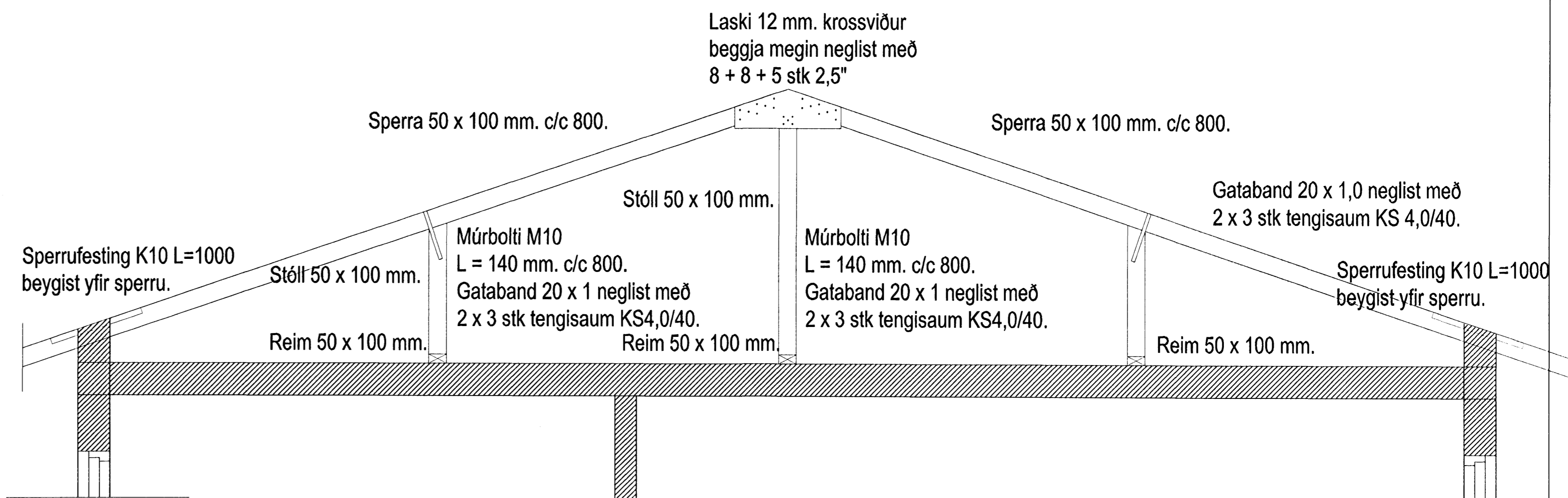
SNID B - B MKV. 1:20.
