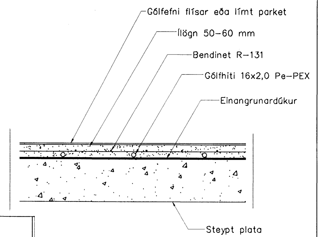
Gólfhiti snið, 1:10
