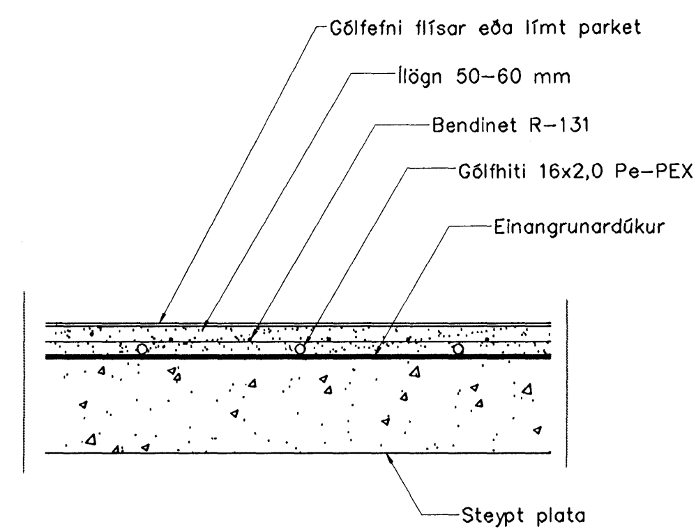
Gólfhiti snið, 1:10
