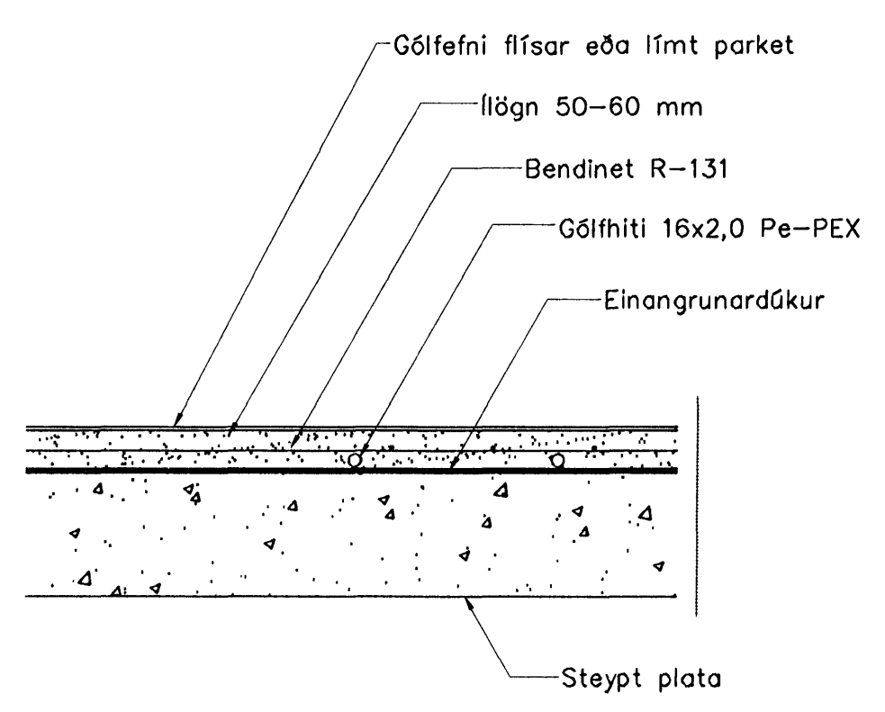
Gólfhiti snið, 1:10
