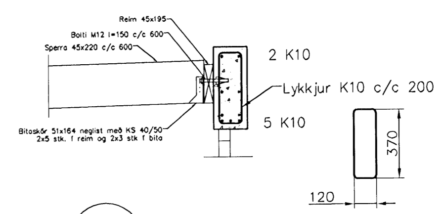
Snið 1 1:20 1-02
