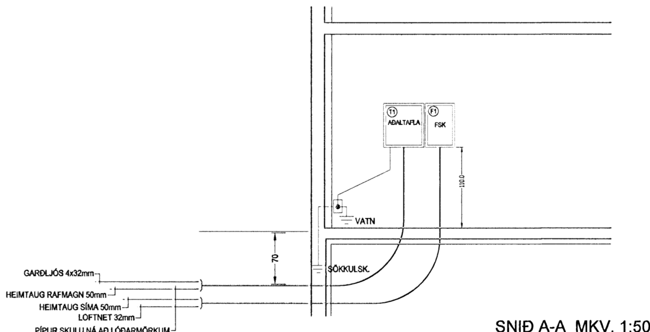
SNID A-A MKV. 1:50
