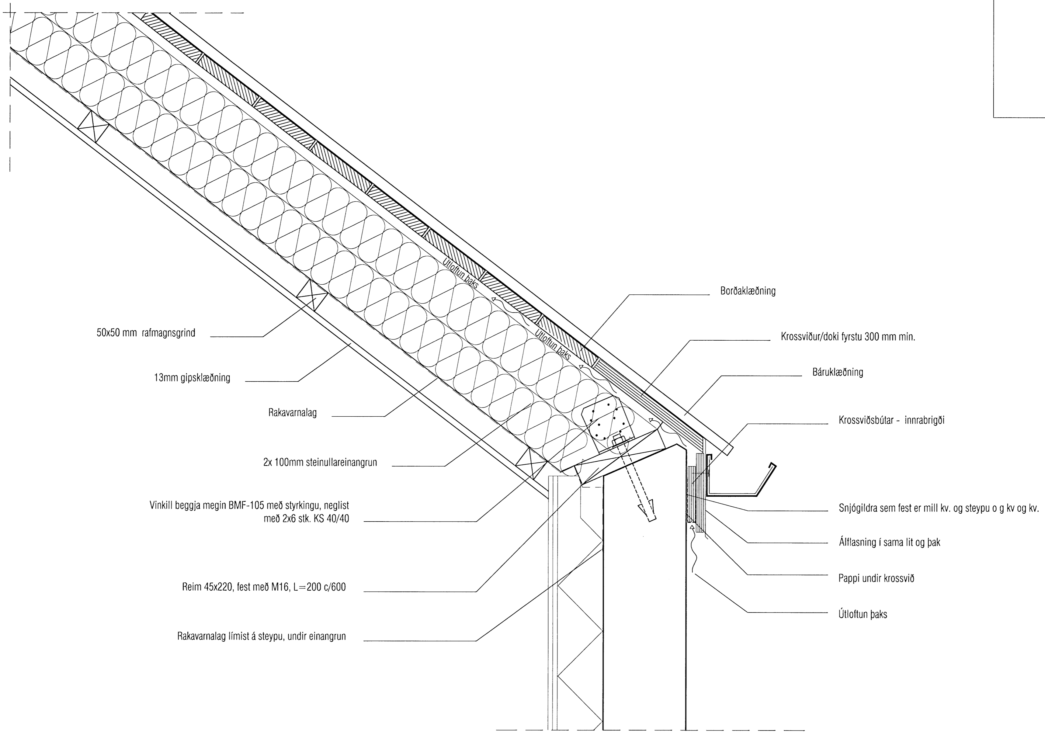
DEILI ÞAKKANTAR - 1:5
