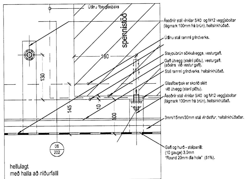
DEILI 02 mkv.1:5 - LÁRÉTT DEILI VIÐ STEYPTA SÖKKULBRÚN - (VESTUR GAFL)
