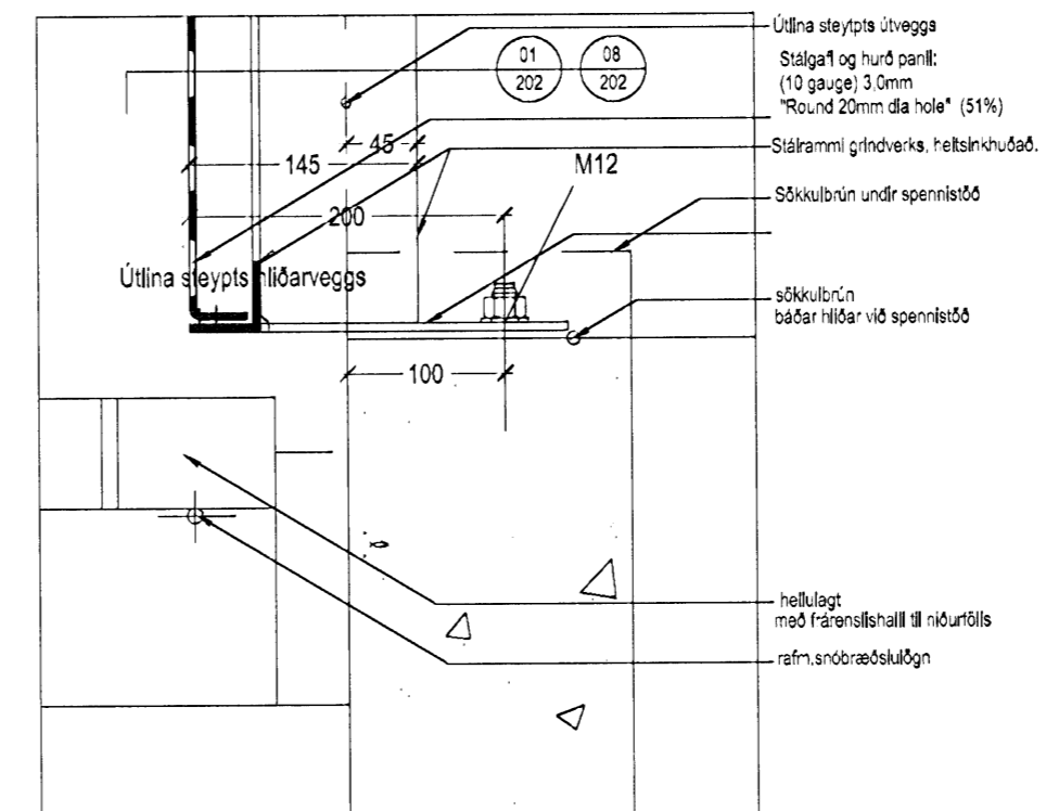
DEILI 06 mkv.1:5 - LÓÐRÉTT DEILI VIÐ SÖKKULBRÚN - (VESTUR GAFL)
