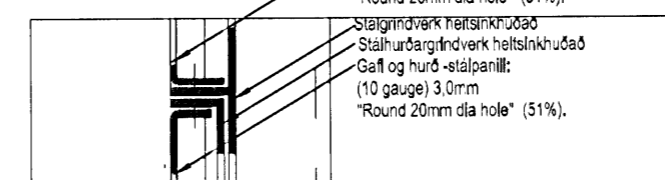
DEILI 05 mkv.1:5 - LÓÐRÉTT DEILI GEGNUM HURÐ Í GAFL GRINDVERK - (VESTUR GAFL)
