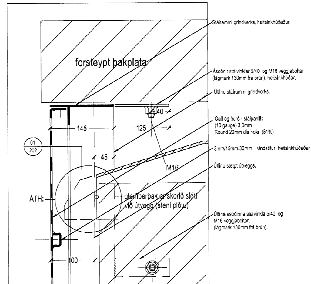
DEILI 04 mkv.1:5 - LÓÐRÉTT DEILI VIÐ NEÐRABORÐ FORSTEYPTS ÞAKS - (VESTUR GAFL)
