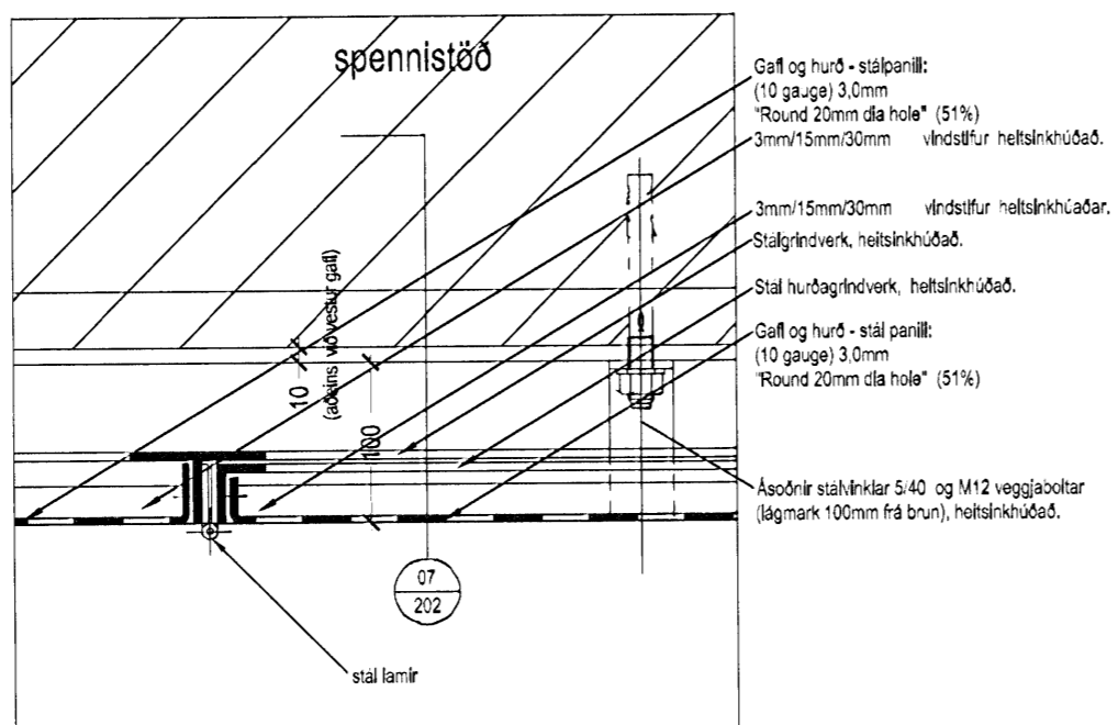
DEILI 03 mkv.1:5 - LÁRÉTT DEILI GEGNUM HURÐ Í GAFL GRINDVERK VIÐ SÖKKULBRÚN - (VESTUR GAFL)
