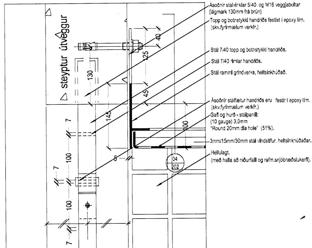
DEILI 01 mkv.1:5 - LÁRÉTT DEILI VIÐ STEYPTAN ÚTVEGG - (VESTUR GAFL)
