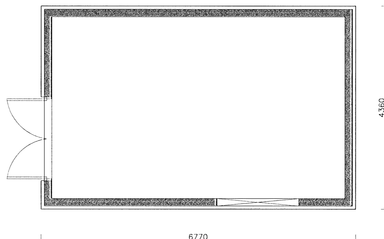
GRUNNMYND EFTIR KLÆDNINGU
