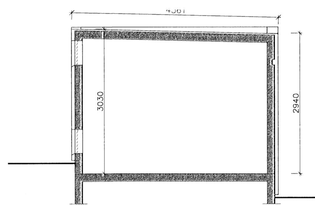
SNIÐ 1:50 EFTIR KLÆÐNINGU
