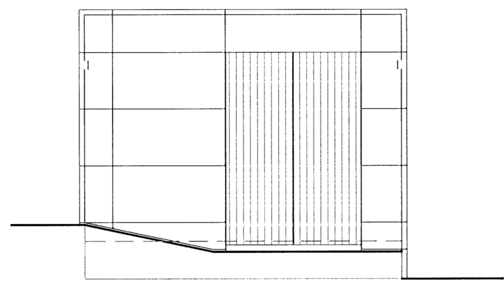
VESTURHLIÐ 1:50 EFTIR KLÆÐNINGU
