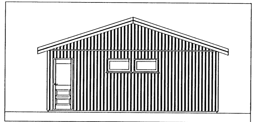
AUSTUR ÚTLIT 1:100
