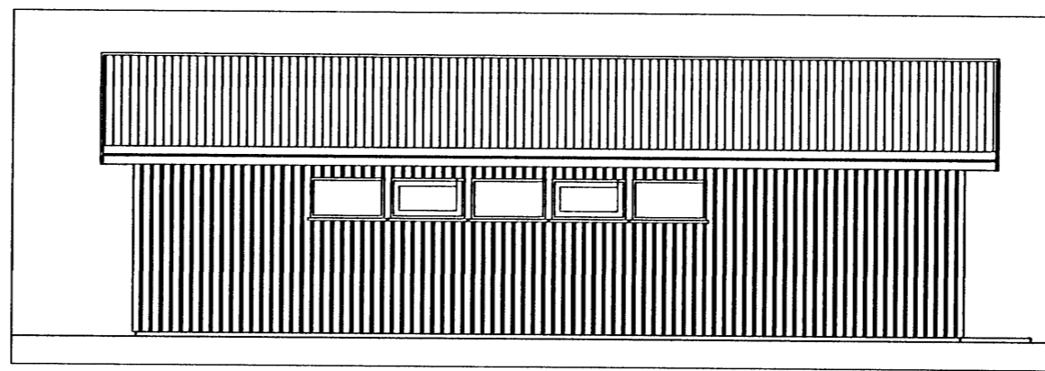
NORÐUR ÚTLIT 1:100
