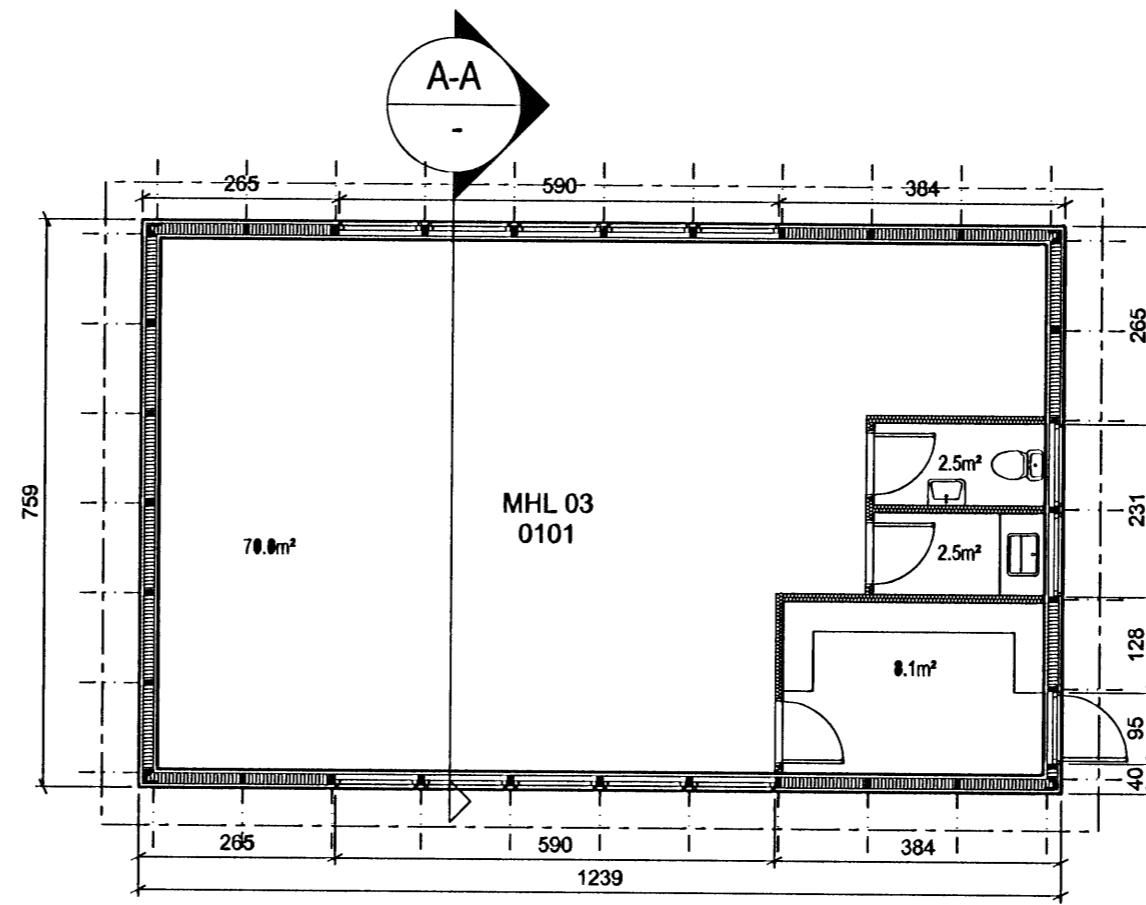
GRUNNMYND 1:100
