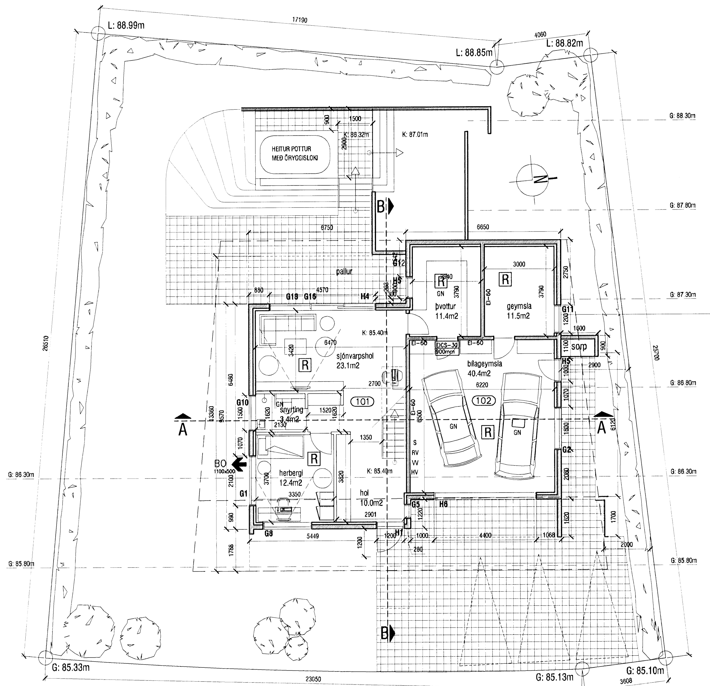
Grunnmynd neðri hæðar mkv. 1:100
