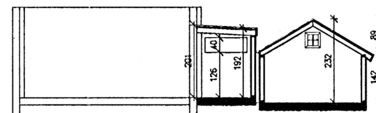
Snið D-D 1:100
