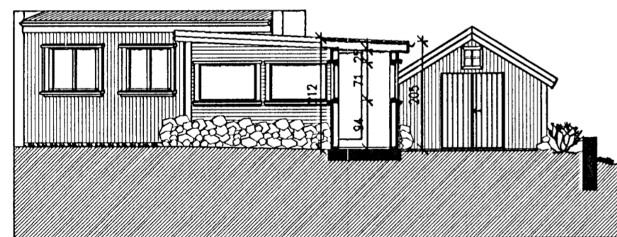
Snið C-C 1:100
