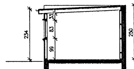
Snið E-E 1:100
