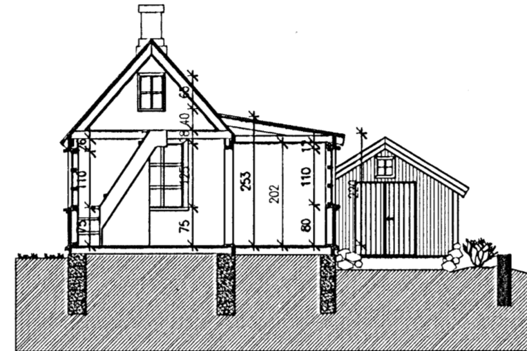
Snið B-B 1:100
