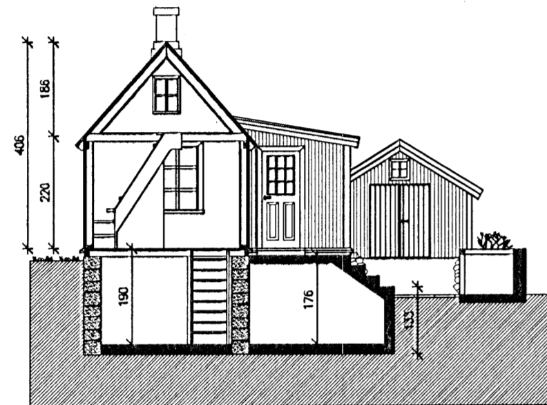
Snið A-A 1:100
