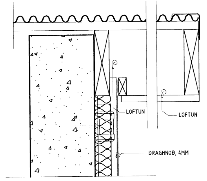
LÓDRÉTT SNIÐ VIÐ ÞAK M.KV. 1 : 5
