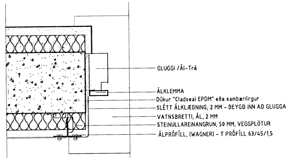
LÁRÉTT SNIÐ VIÐ GLUGGA M.KV. 1 : 5
