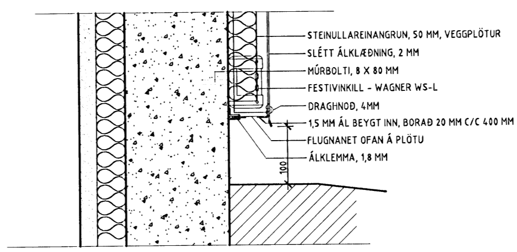
LÓDRÉTT SNIÐ VIÐ JÖRÐ M.KV. 1 : 5
