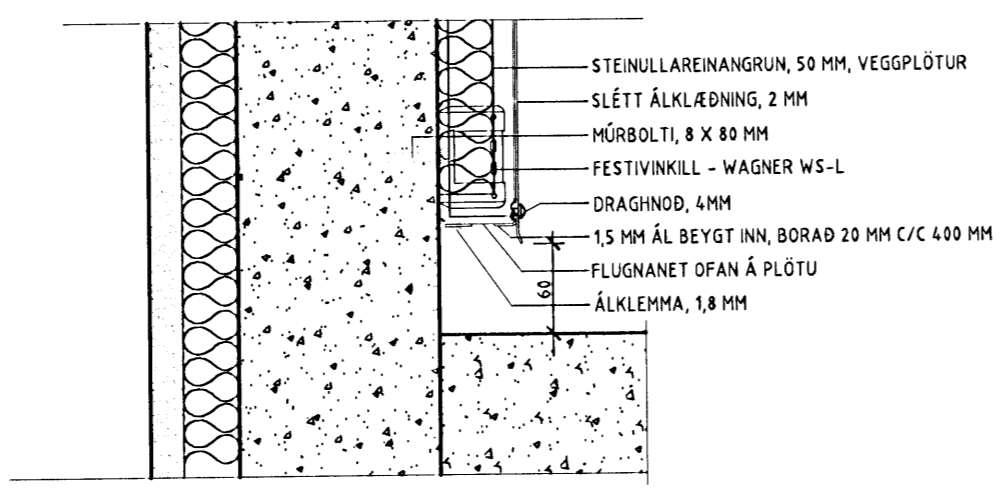
LÓDRÉTT SNIÐ VIÐ SVALGÓLF M.KV. 1 : 5
