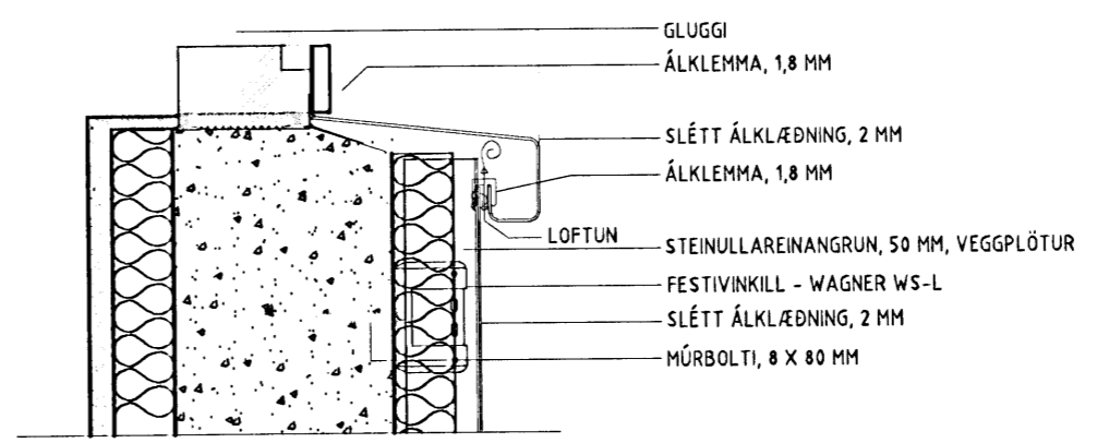
LÓDRÉTT SNIÐ VIÐ GLUGGA M.KV. 1 : 5
