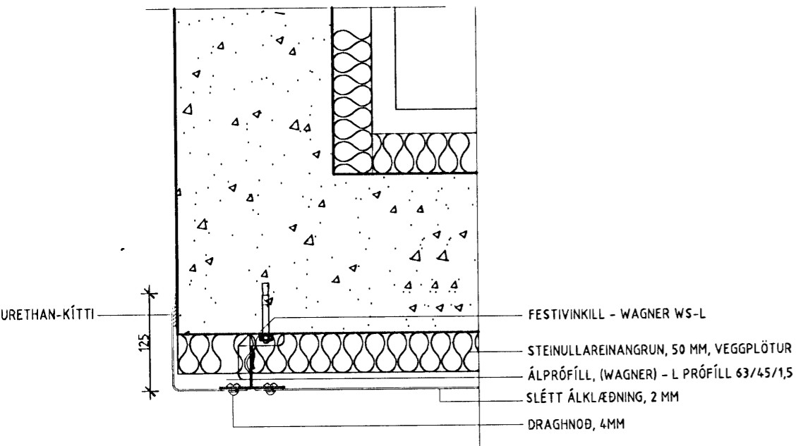
LÁRÉTT SNIÐ ÚTHORN M.KV. 1 : 5
