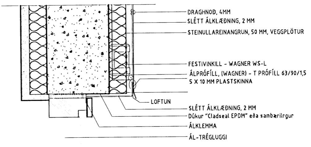
LÓDRÉTT SNIÐ VIÐ GLUGGA M.KV. 1 : 5
