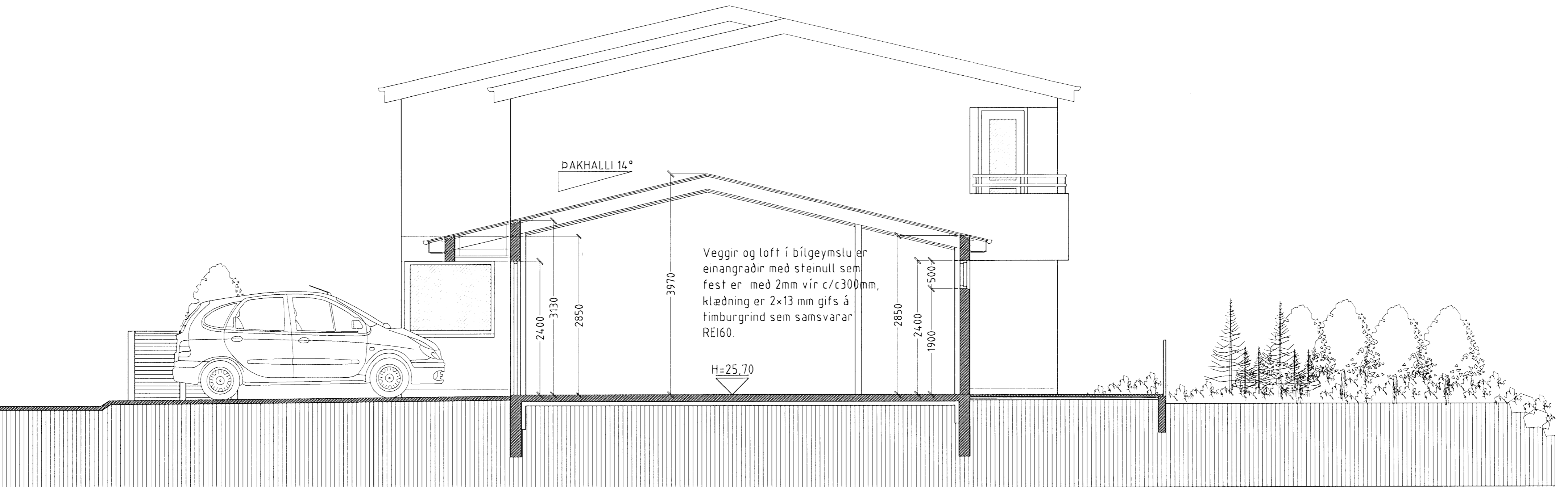
SNID B-B MKV. 1:50.
