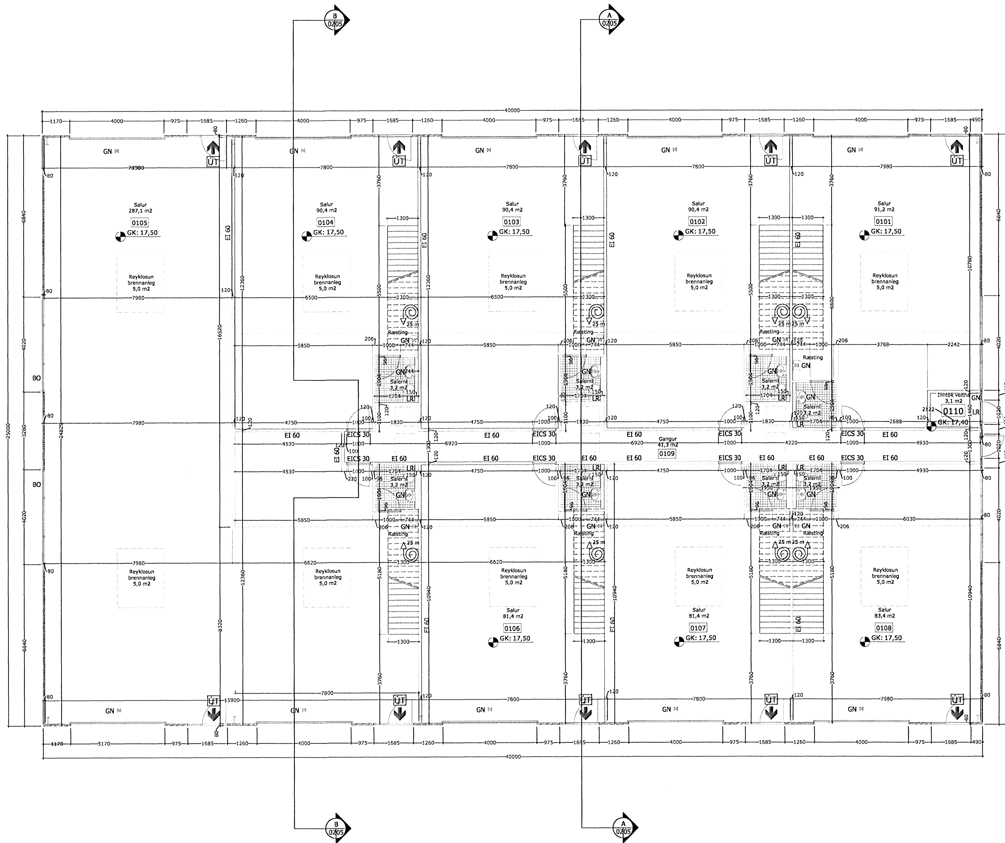
Grunnmynd 1. hæðar 1:100
