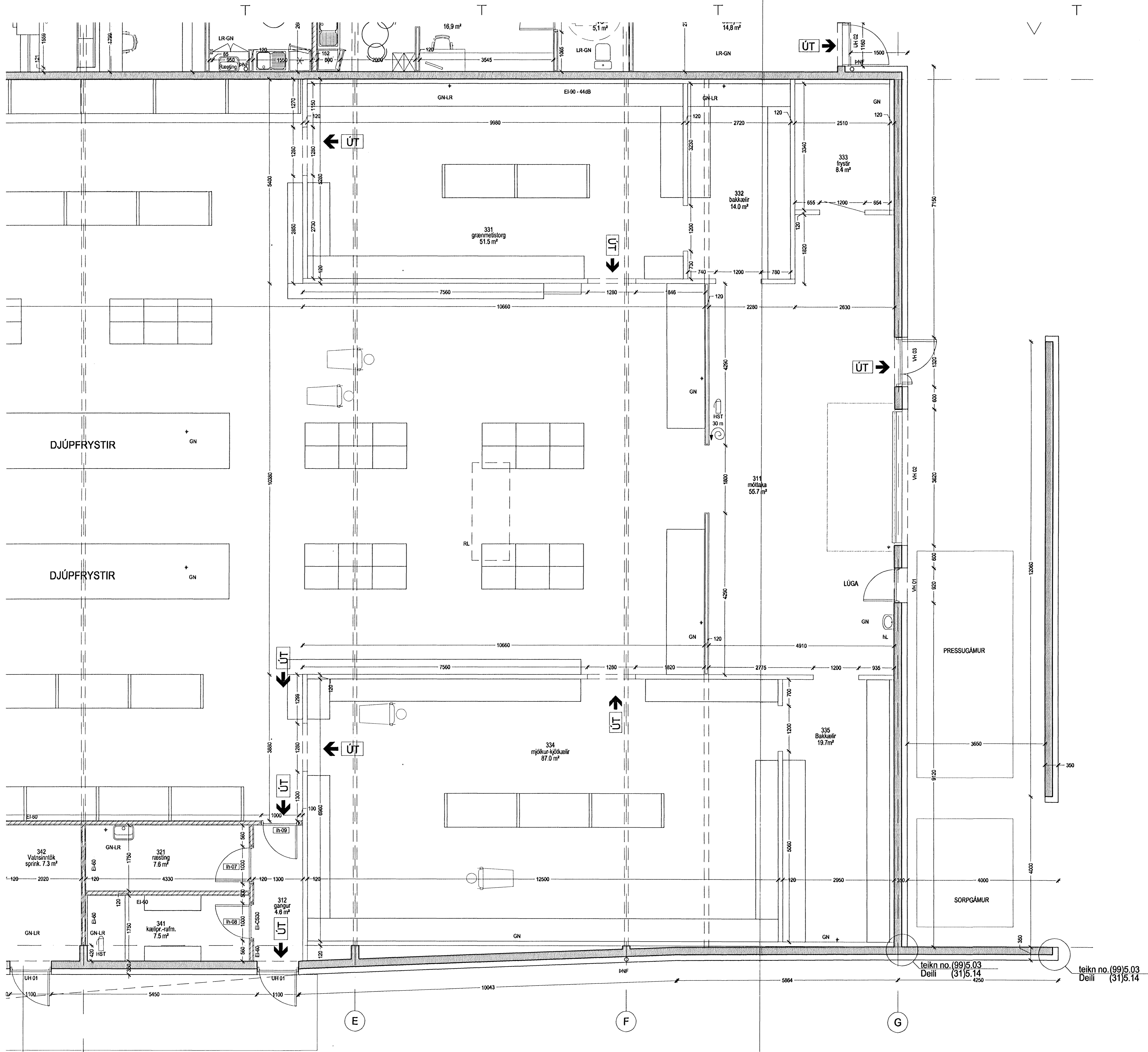
Snið AA D Grunnmynd, modull D-G mkv.1:50
