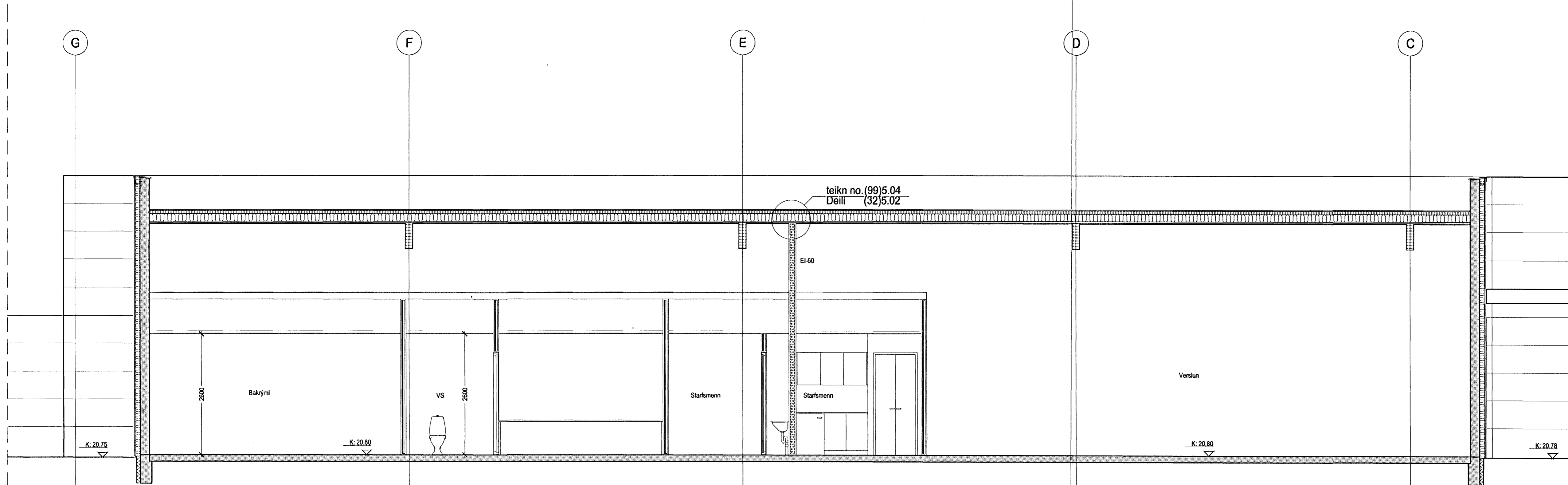
Snið B-B mkv.1:50
