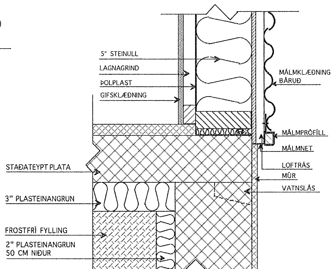
Lóðrétt snið í undir- stk. glugga
