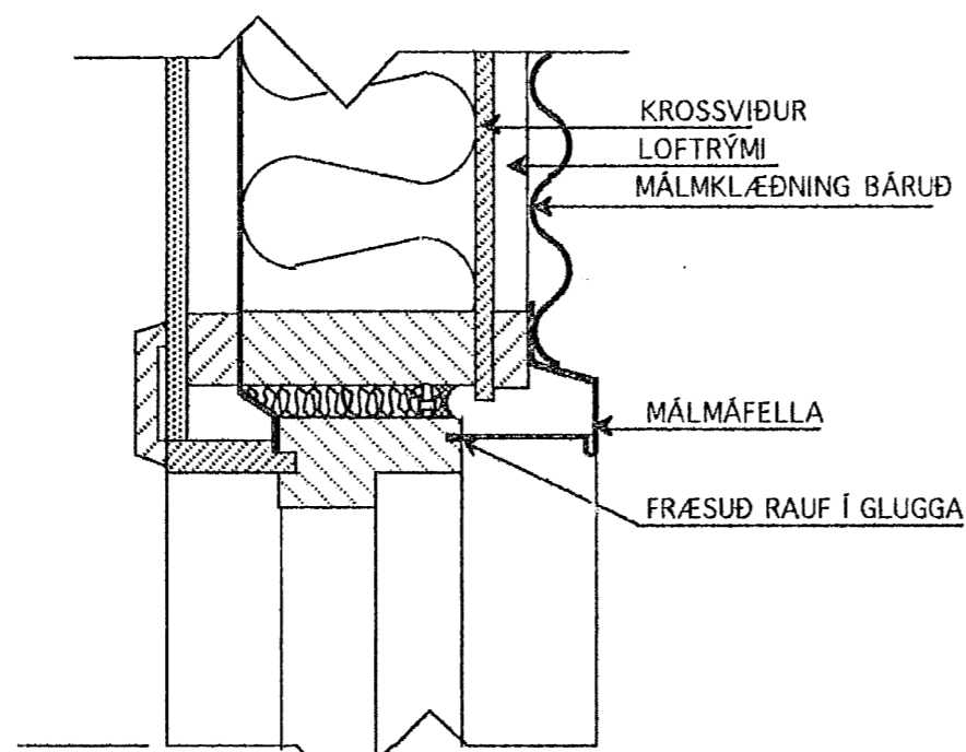
Lárétt snið í yfir- stk. glugga
