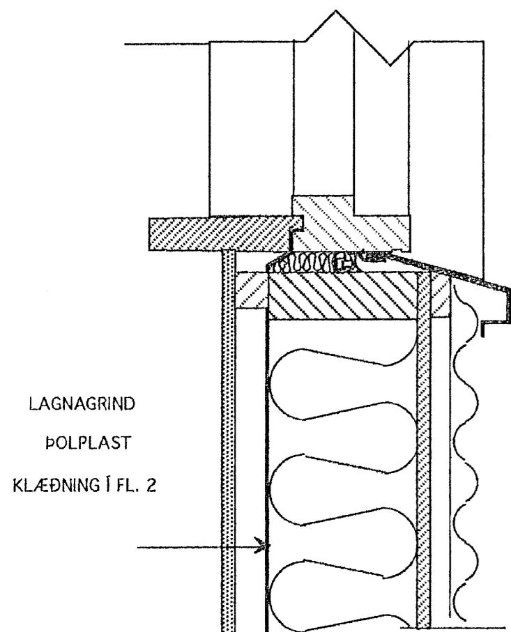
Lóðrétt snið í undir- stk. glugga
