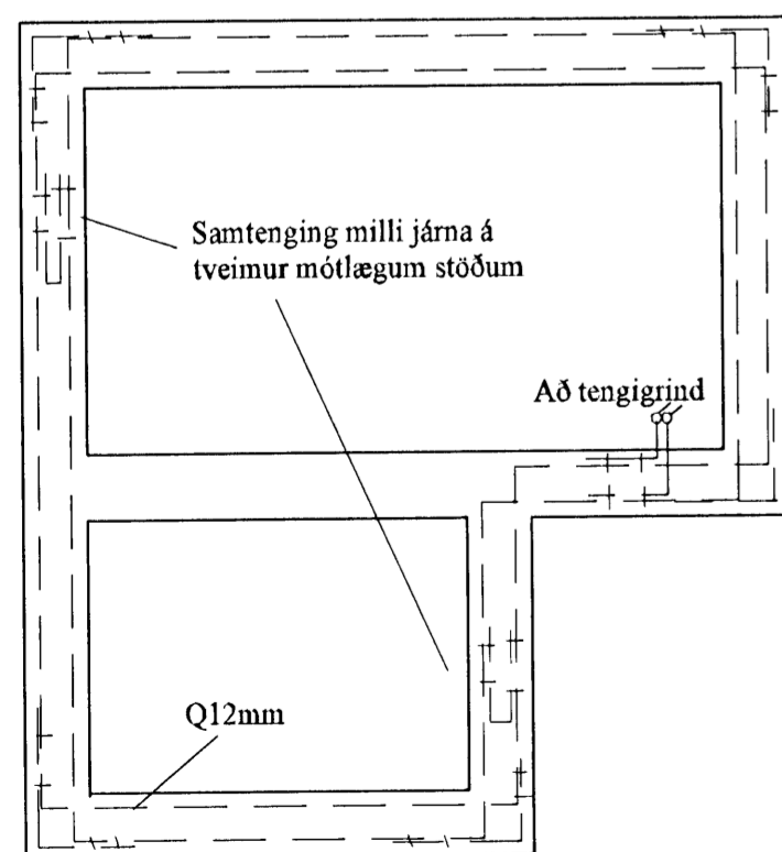
Grunnmynd sökkulveggia
