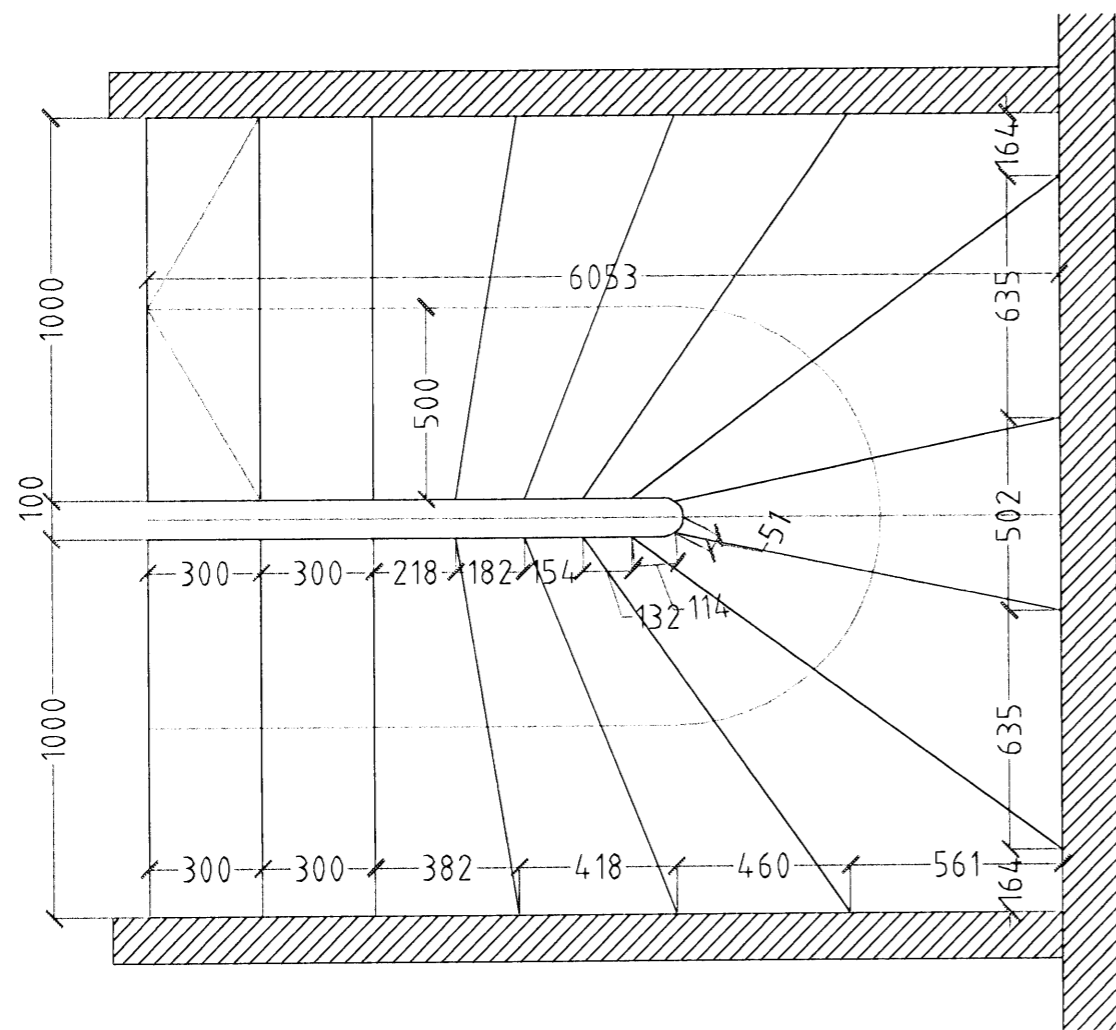
GRUNNMYND STIGI HÚS nr 50 og 52 M. 1:20
