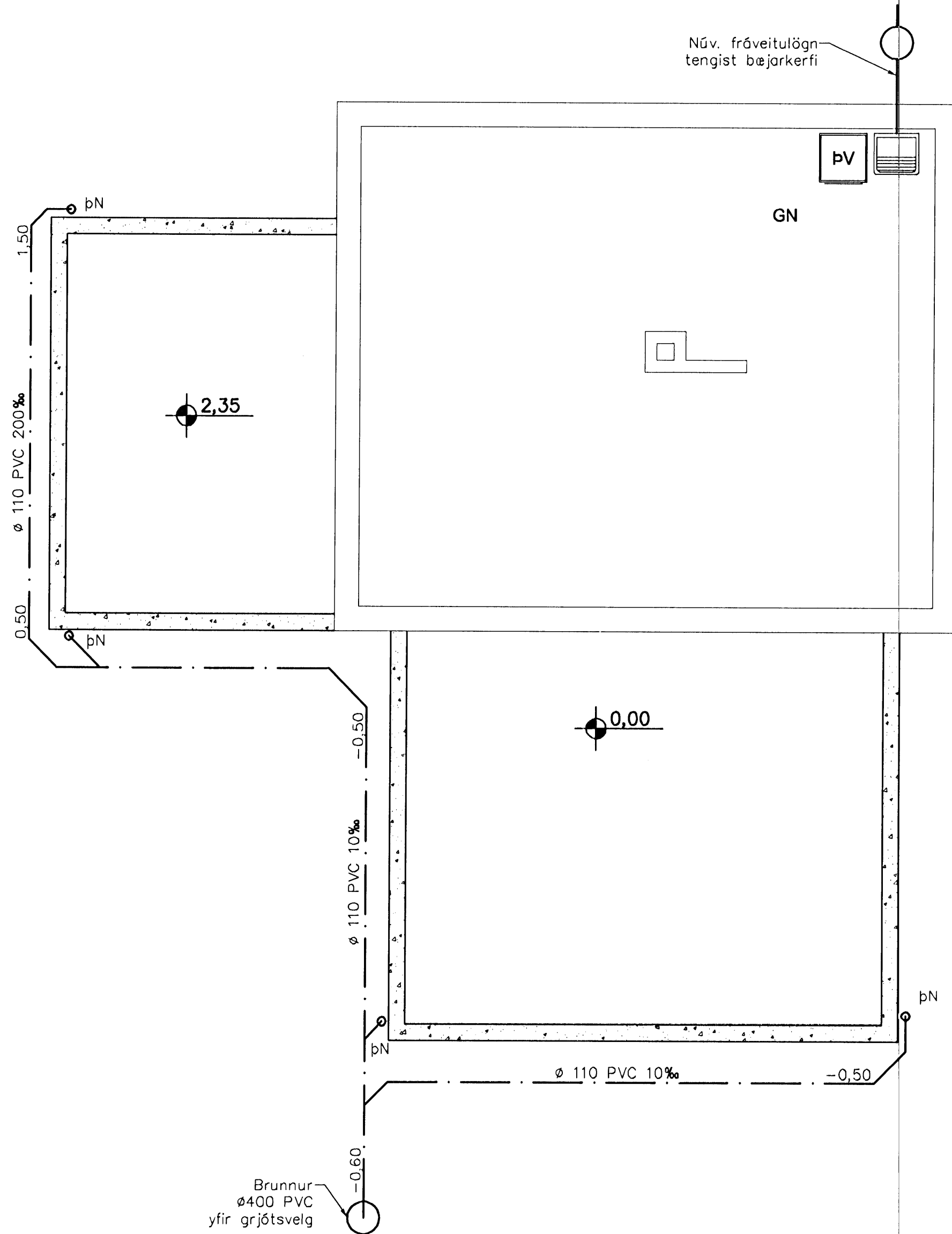
Grunnlagnir 1:50
