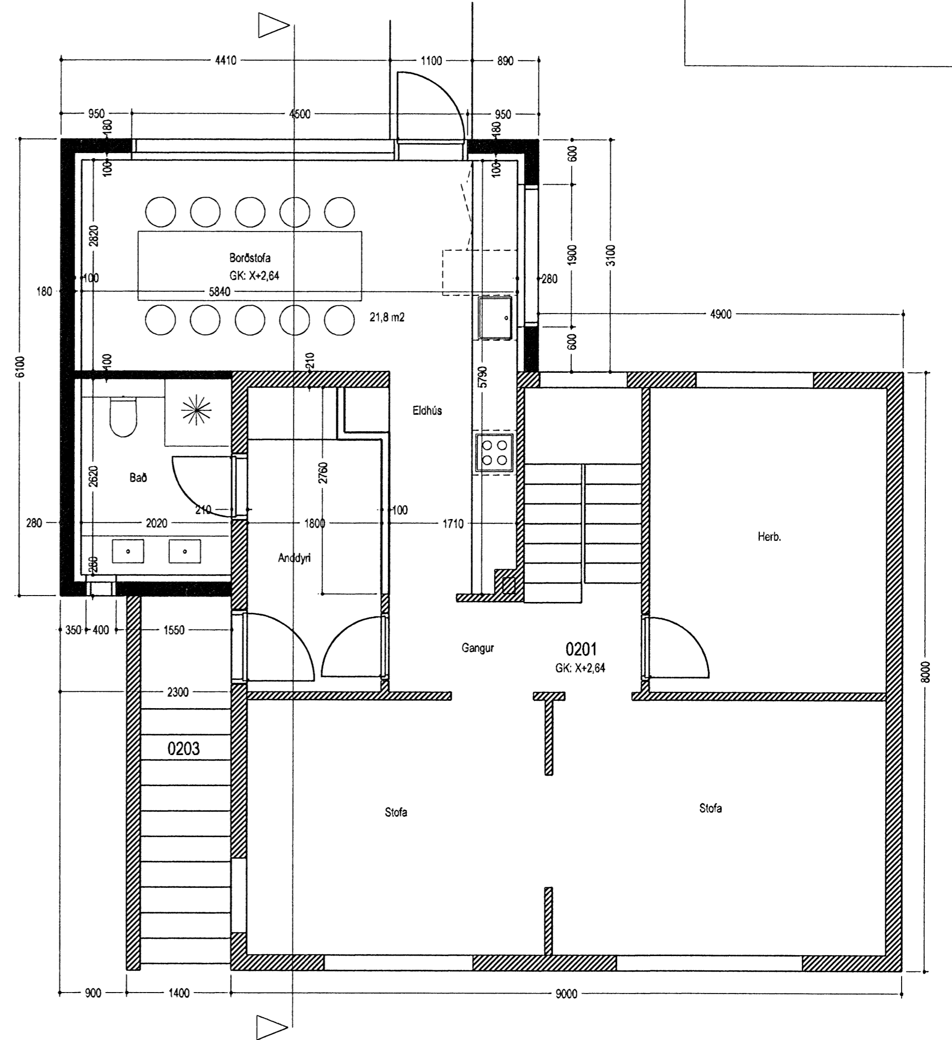
Grunnmynd efri hæðar
