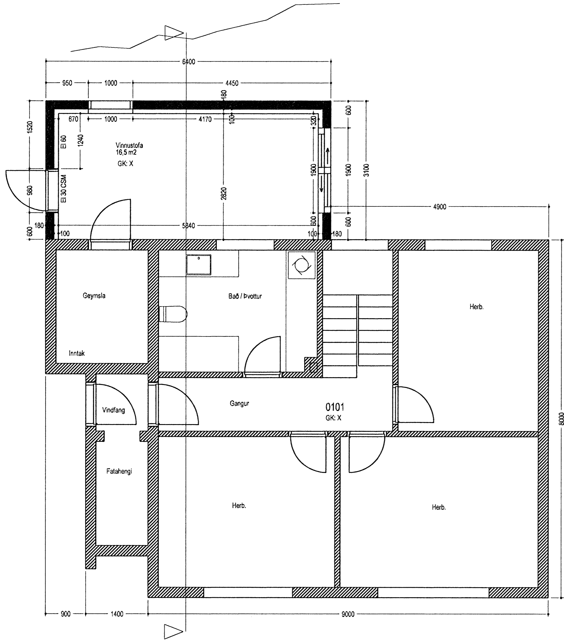
Grunnmynd neðri hæðar
