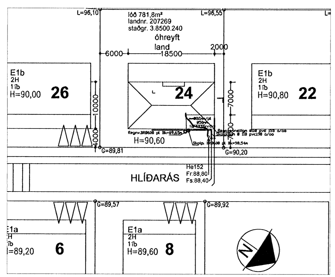
Afstöðumynd Mkv 1:500
