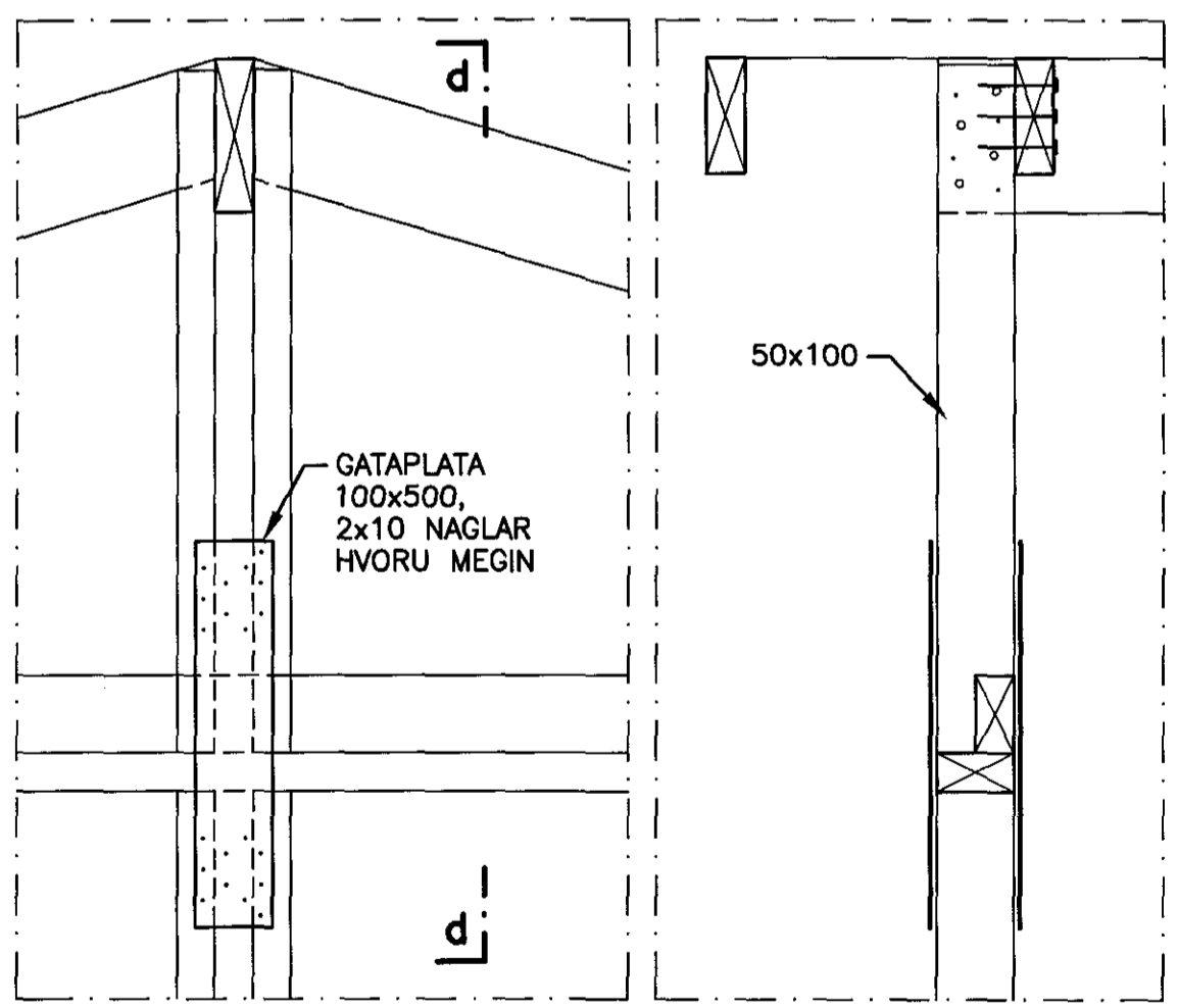
c DEILI MKV. 2
