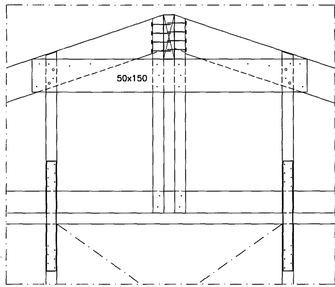
MÁNISBITI Í VEGG YFIR OPI MKV. 2
