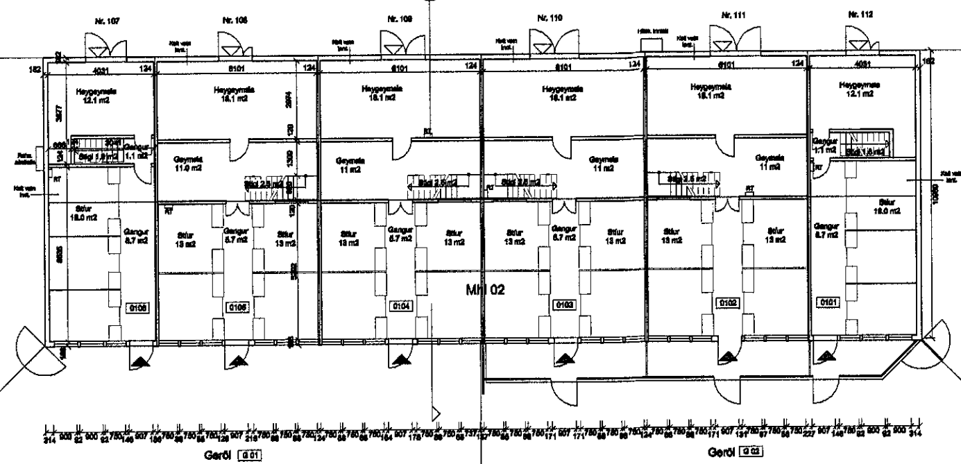
Grunnmynd jarðhæðar 1:100
