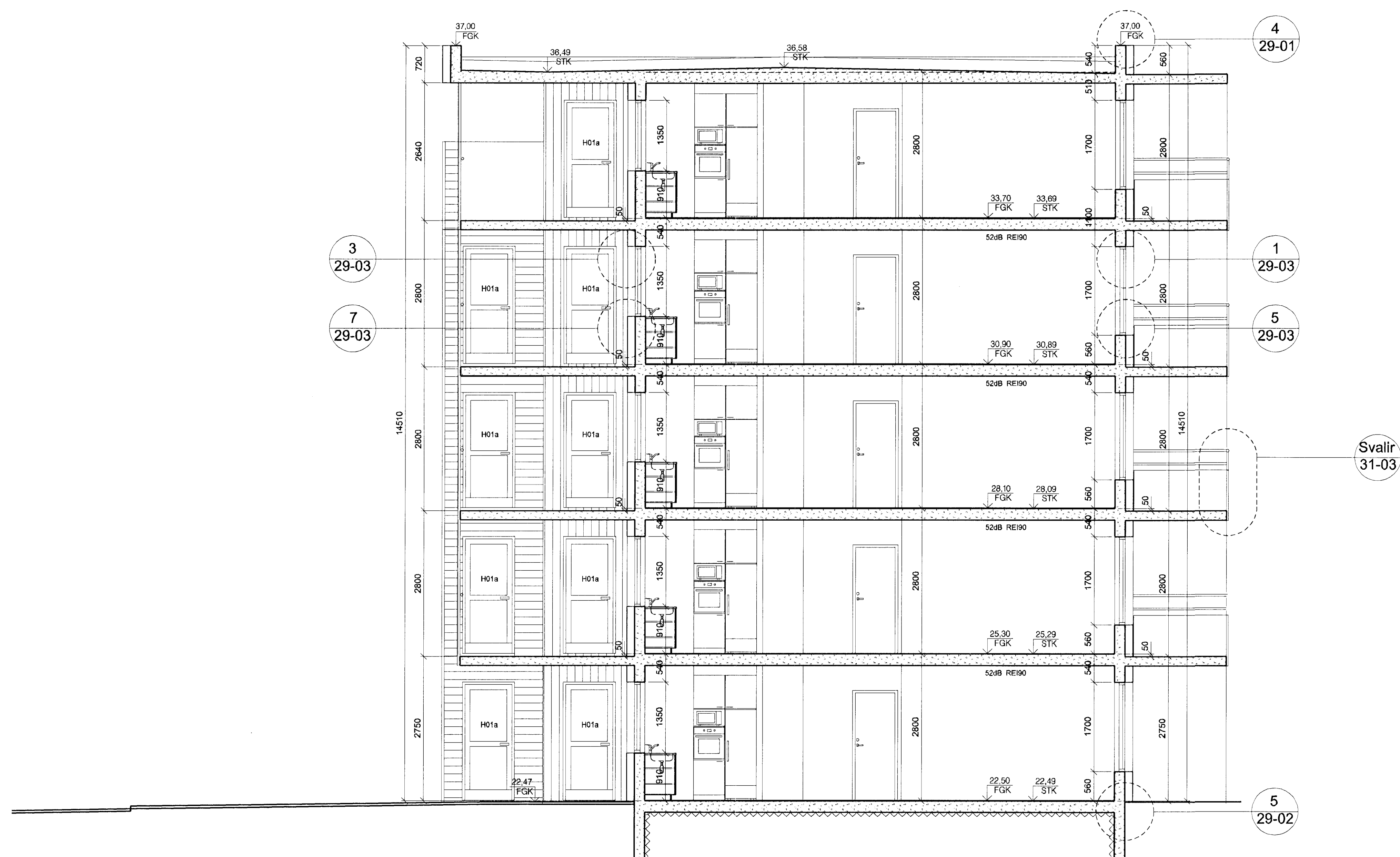
G-G 20-02 20-04 20-06 20-08 20-10 20-12 20-14 SNEIÐING 1:50
