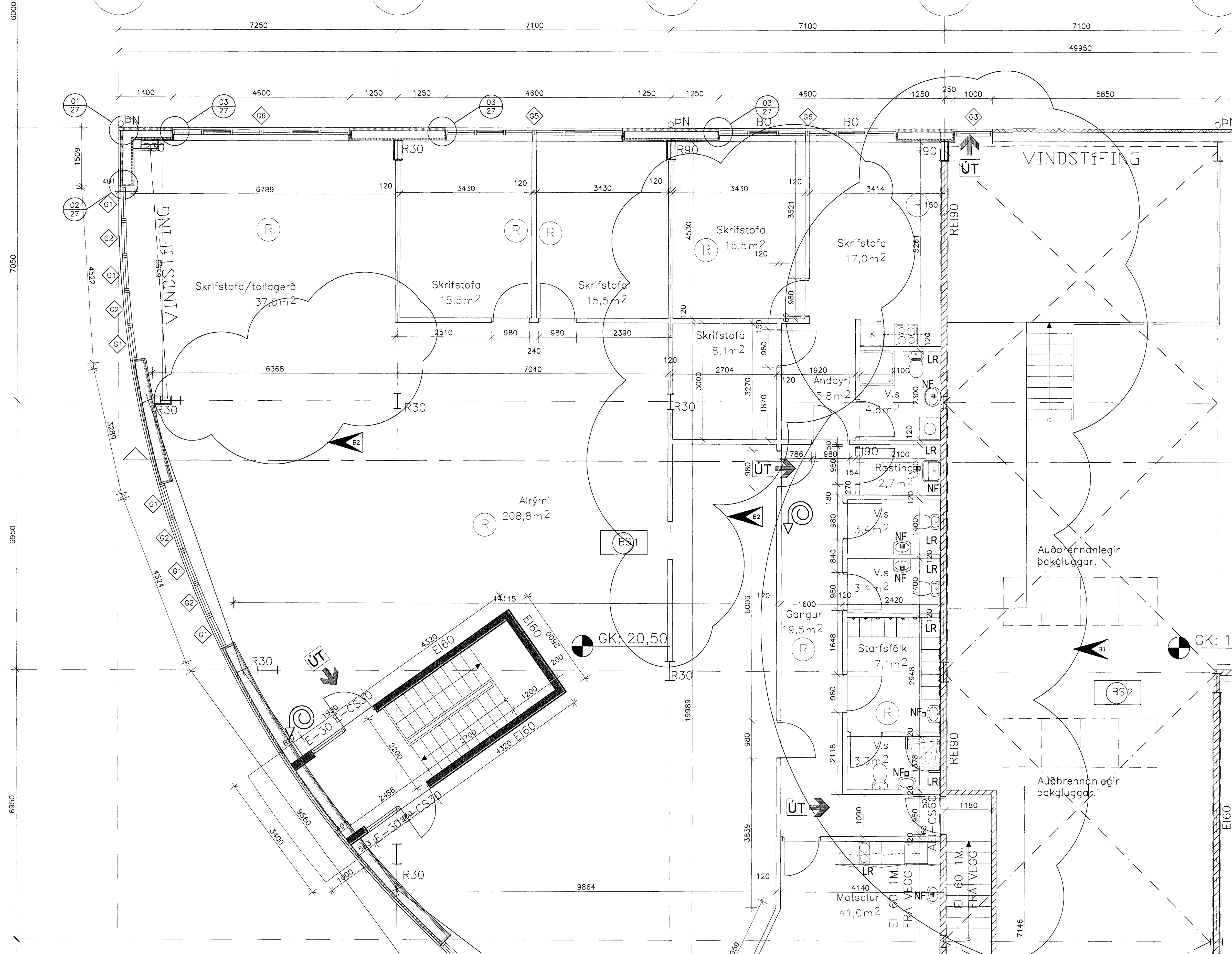
GRUNNMYND 2. HÆÐAR 1:50
