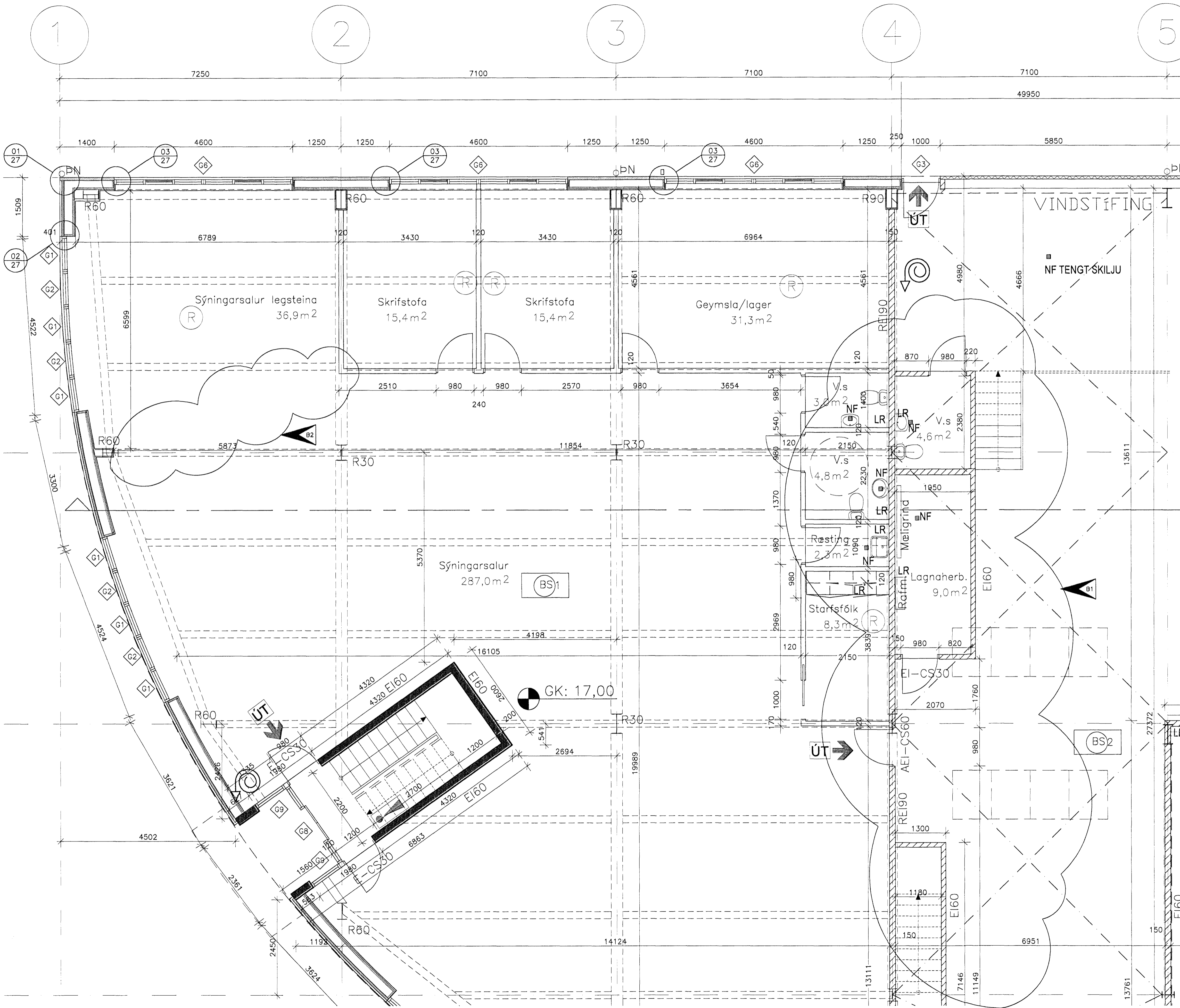
GRUNNMÝND 1. HÆÐAR 1:50
