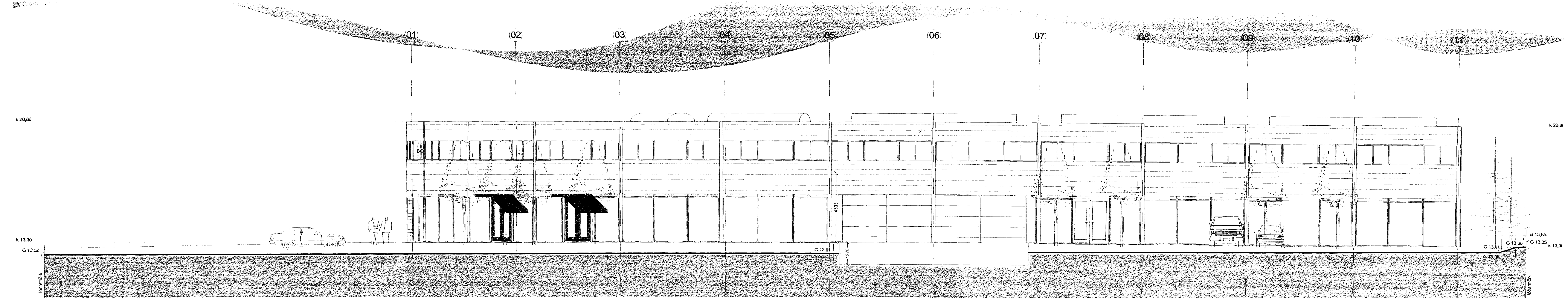
ÚTLIT VESTUR M 1 : 100
