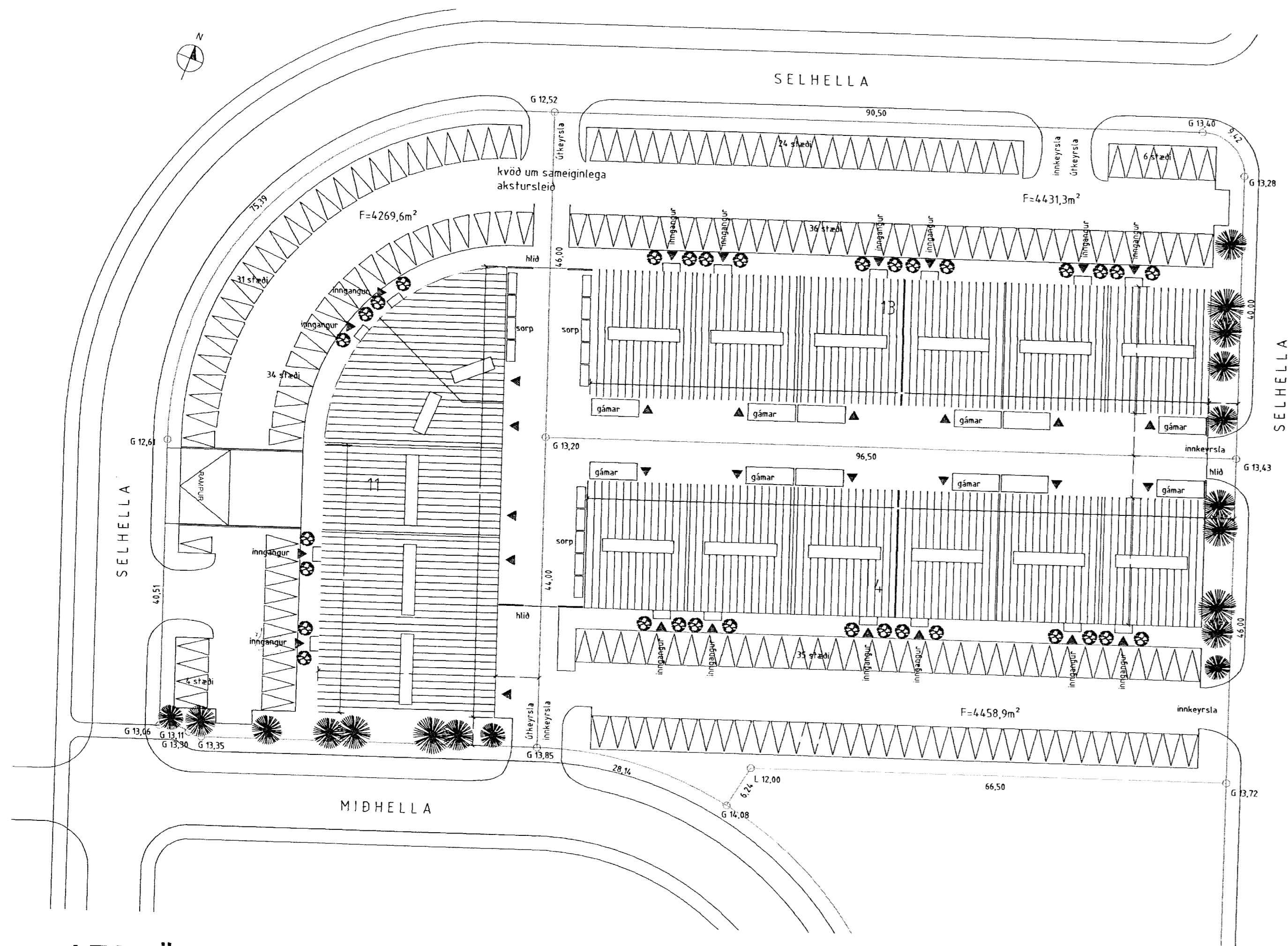
AFSTÖÐUMYND M. 1 : 500.
