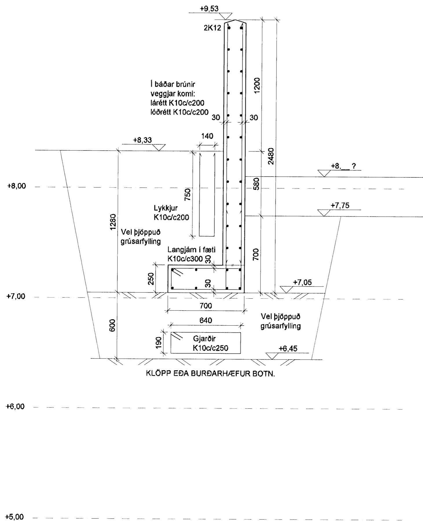
I 02 03 SNIÐ M. 1:20
