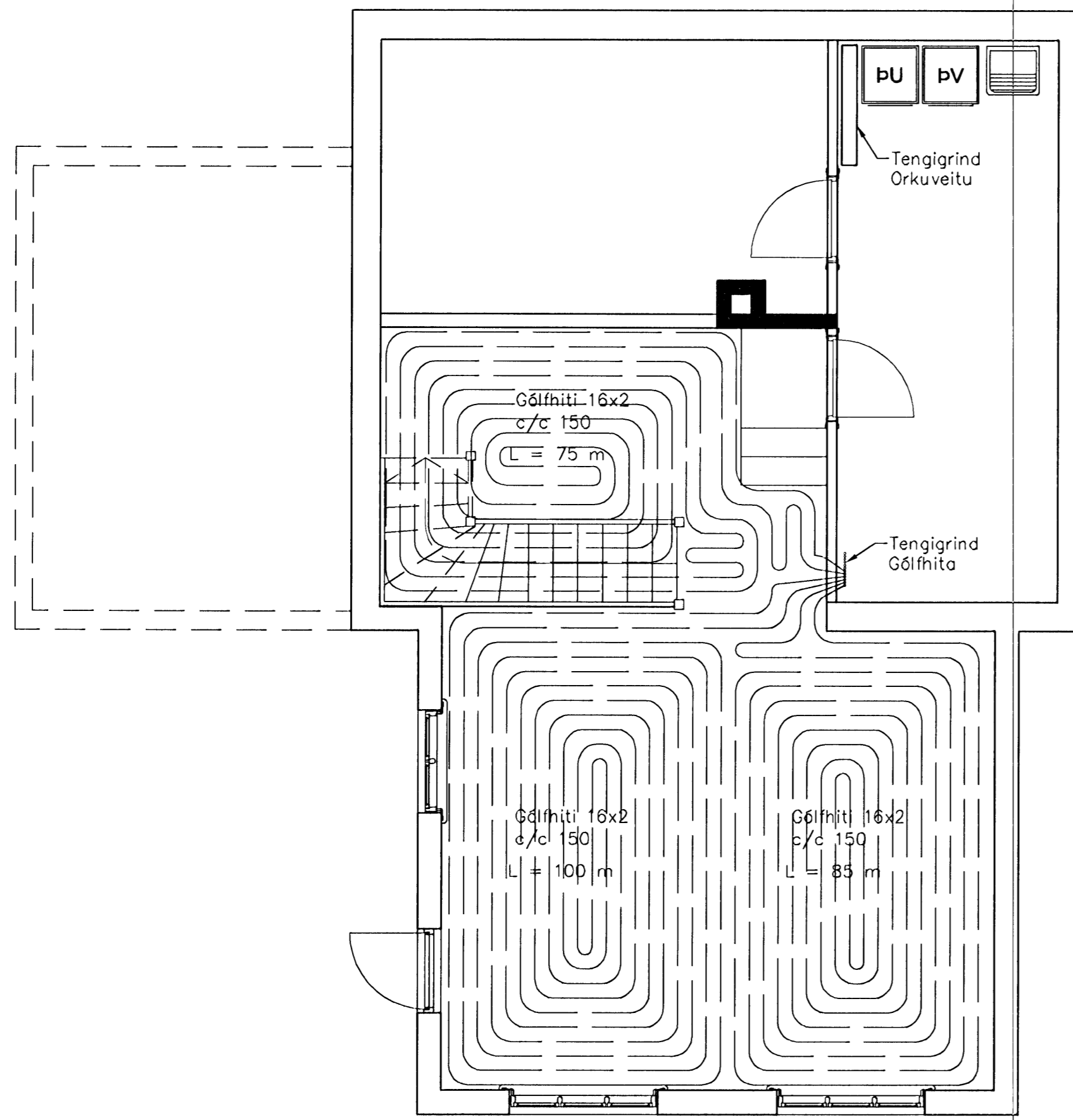
Gólfhiti kjallara, 1:50
